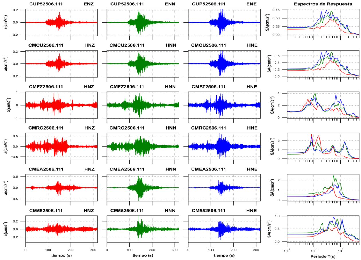
Figura 3d. Acelerogramas registrados y espectros de respuesta estimados para los registros obtenidos durante el sismo del 11 de junio de 2025 (M4.7)
