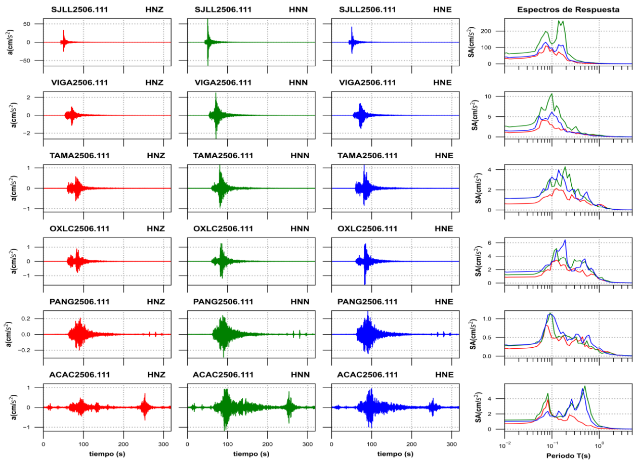
Figura 3a. Acelerogramas registrados y espectros de respuesta estimados para los registros obtenidos durante el sismo del 11 de junio de 2025 (M4.7)
