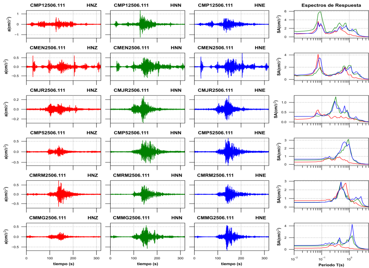
Figura 3c. Acelerogramas registrados y espectros de respuesta estimados para los registros obtenidos durante el sismo del 11 de junio de 2025 (M4.7)
