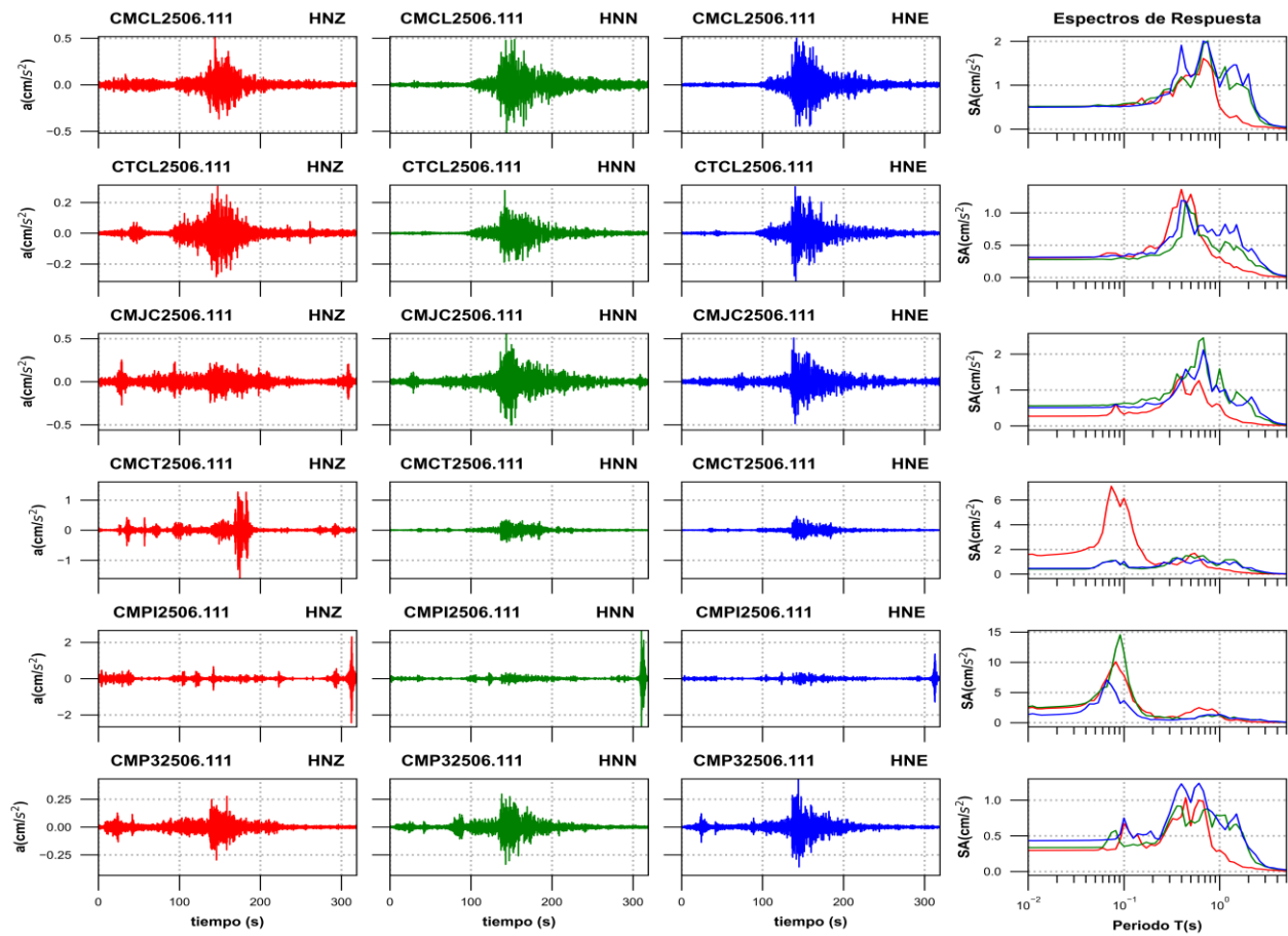
Figura 3f. Acelerogramas registrados y espectros de respuesta estimados para los registros obtenidos durante el sismo del 11 de junio de 2025 (M4.7)
