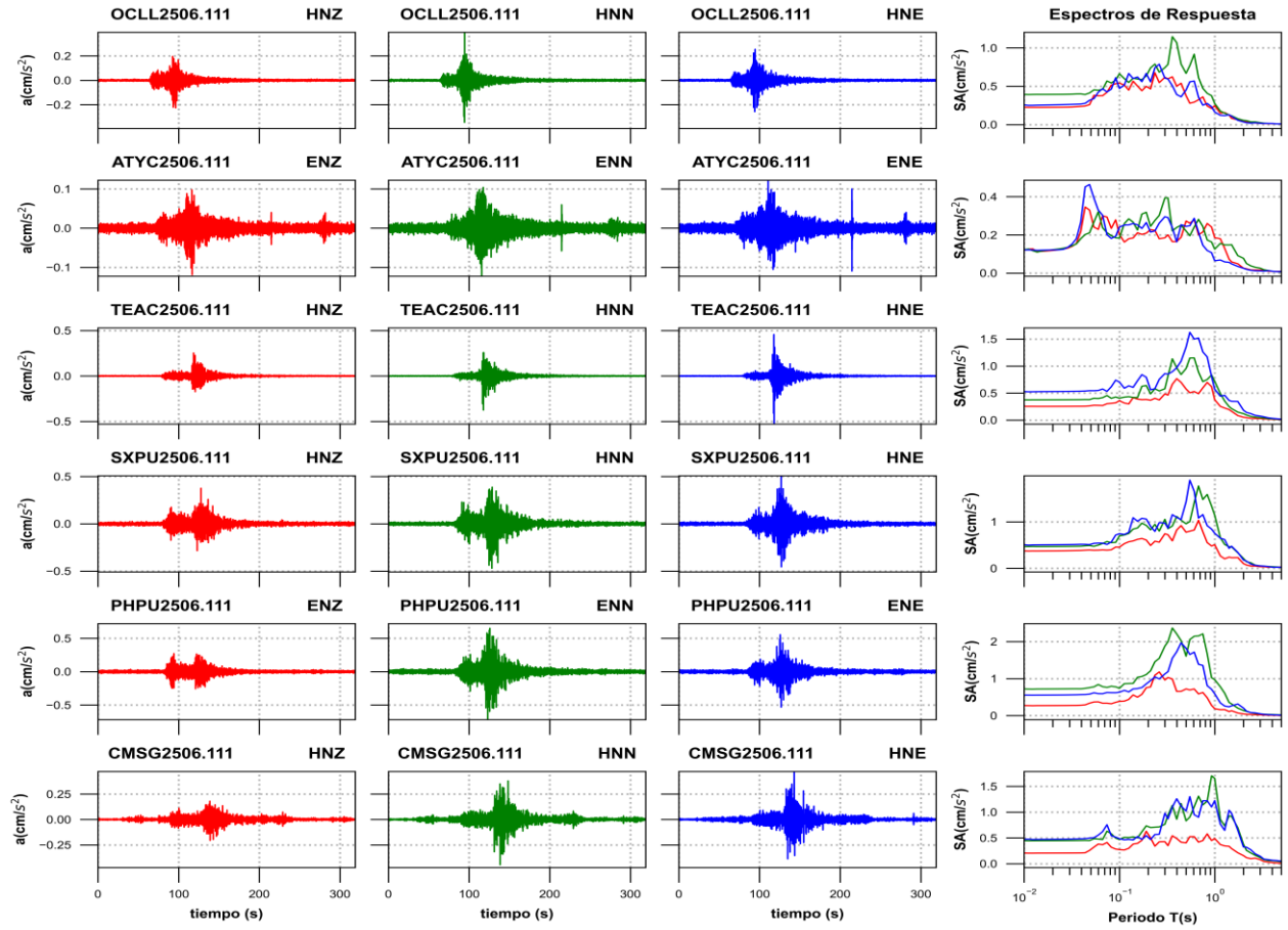
Figura 3b. Acelerogramas registrados y espectros de respuesta estimados para los registros obtenidos durante el sismo del 11 de junio de 2025 (M4.7)
