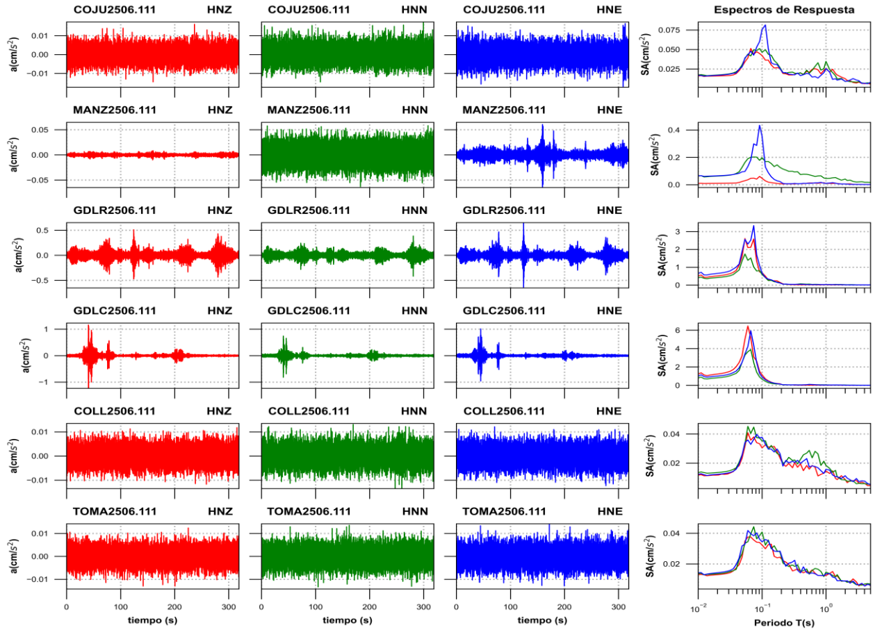
Figura 3h. Acelerogramas registrados y espectros de respuesta estimados para los registros obtenidos durante el sismo del 11 de junio de 2025 (M4.7)
