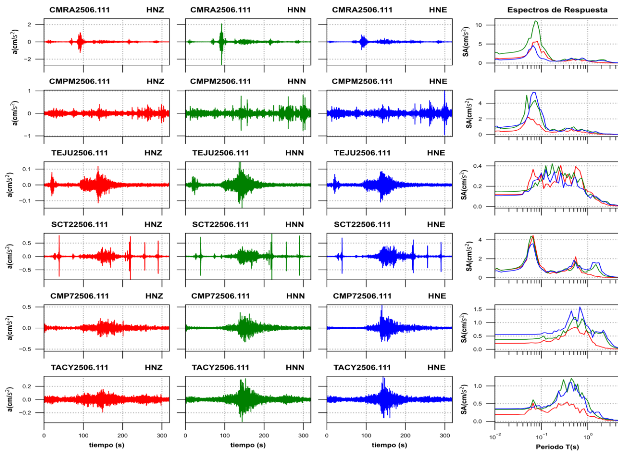
Figura 3e. Acelerogramas registrados y espectros de respuesta estimados para los registros obtenidos durante el sismo del 11 de junio de 2025 (M4.7)
