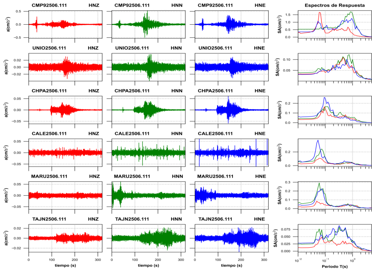
Figura 3g. Acelerogramas registrados y espectros de respuesta estimados para los registros obtenidos durante el sismo del 11 de junio de 2025 (M4.7)
