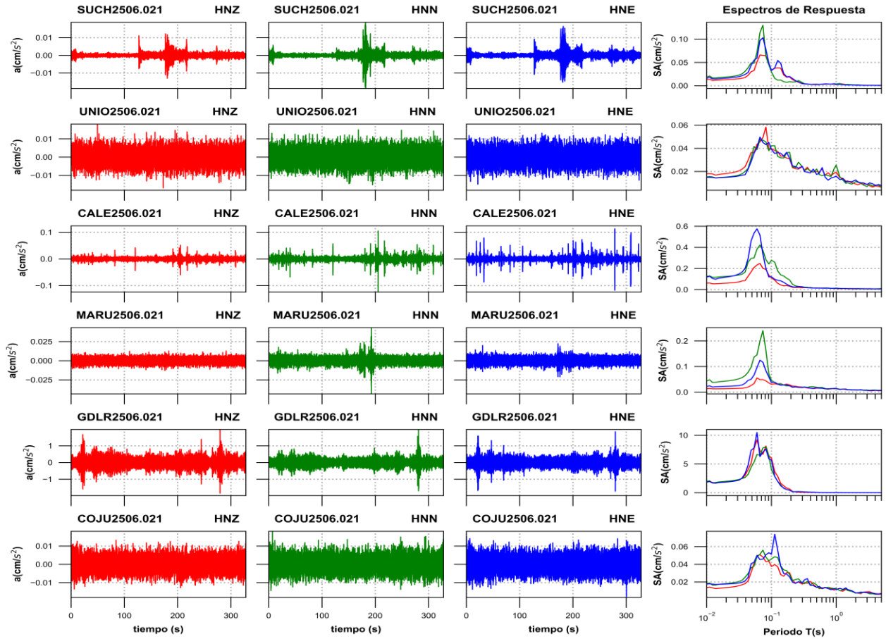
Figura 3h. Acelerogramas registrados y espectros de respuesta estimados para los registros obtenidos durante el sismo del 02 de junio de 2025 (M4.9)
