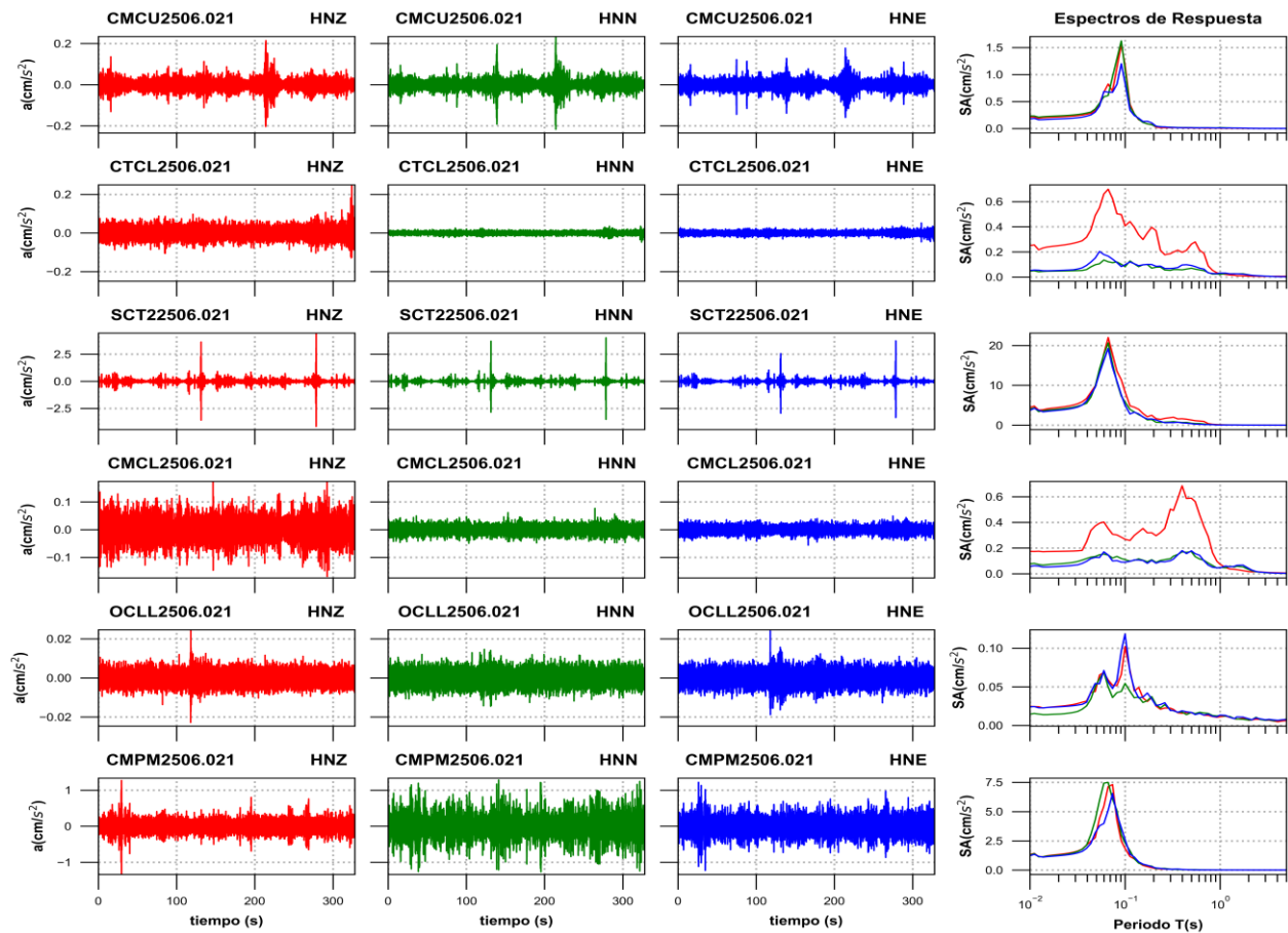
Figura 3f. Acelerogramas registrados y espectros de respuesta estimados para los registros obtenidos durante el sismo del 02 de junio de 2025 (M4.9)
