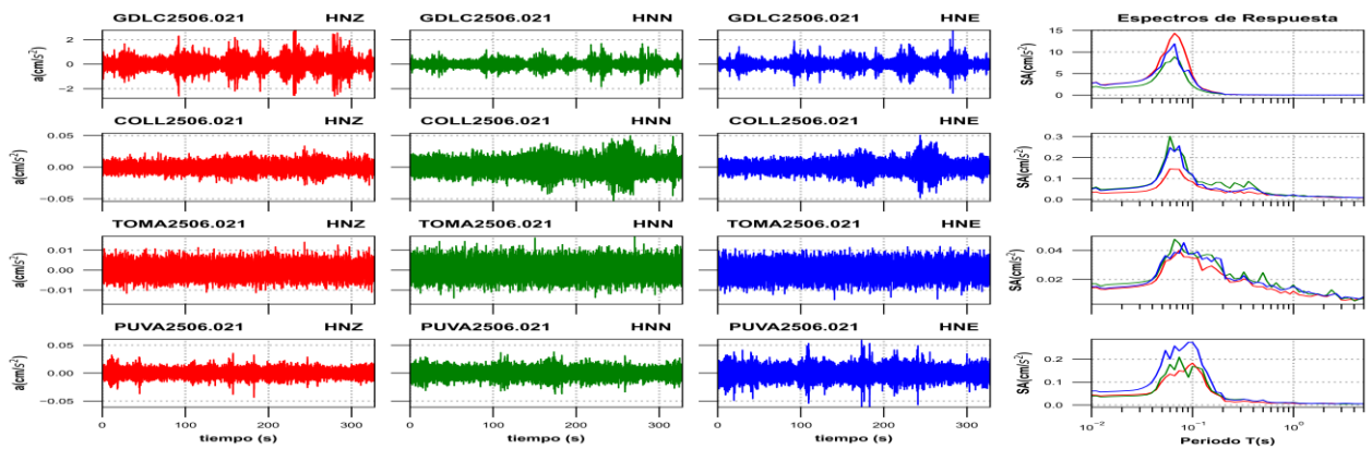
Figura 3i. Acelerogramas registrados y espectros de respuesta estimados para los registros obtenidos durante el sismo del 02 de junio de 2025 (M4.9)
