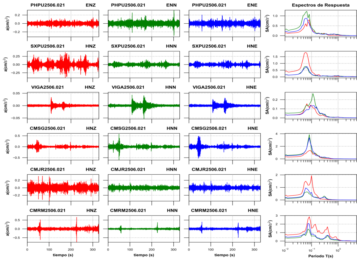
Figura 3b. Acelerogramas registrados y espectros de respuesta estimados para los registros obtenidos durante el sismo del 02 de junio de 2025 (M4.9)
