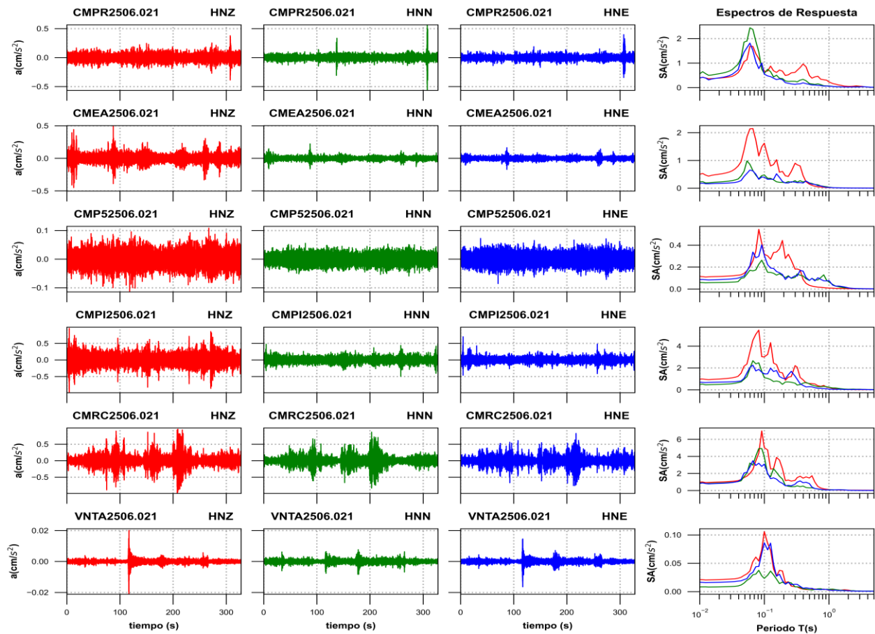
Figura 3d. Acelerogramas registrados y espectros de respuesta estimados para los registros obtenidos durante el sismo del 02 de junio de 2025 (M4.9)
