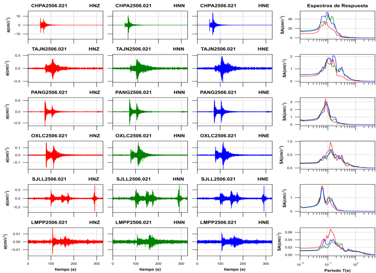
Figura 3a. Acelerogramas registrados y espectros de respuesta estimados para los registros obtenidos durante el sismo del 02 de junio de 2025 (M4.9)
