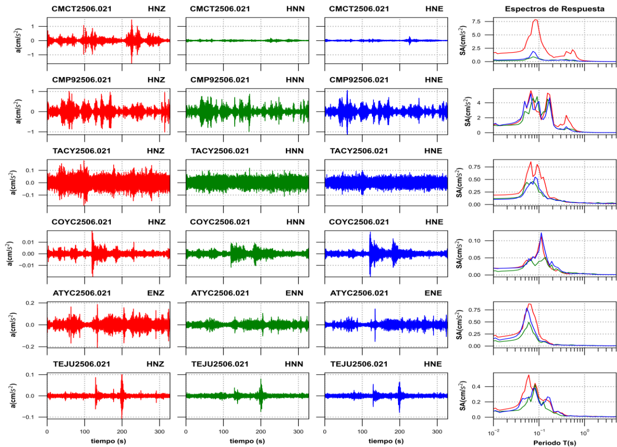
Figura 3g. Acelerogramas registrados y espectros de respuesta estimados para los registros obtenidos durante el sismo del 02 de junio de 2025 (M4.9)
