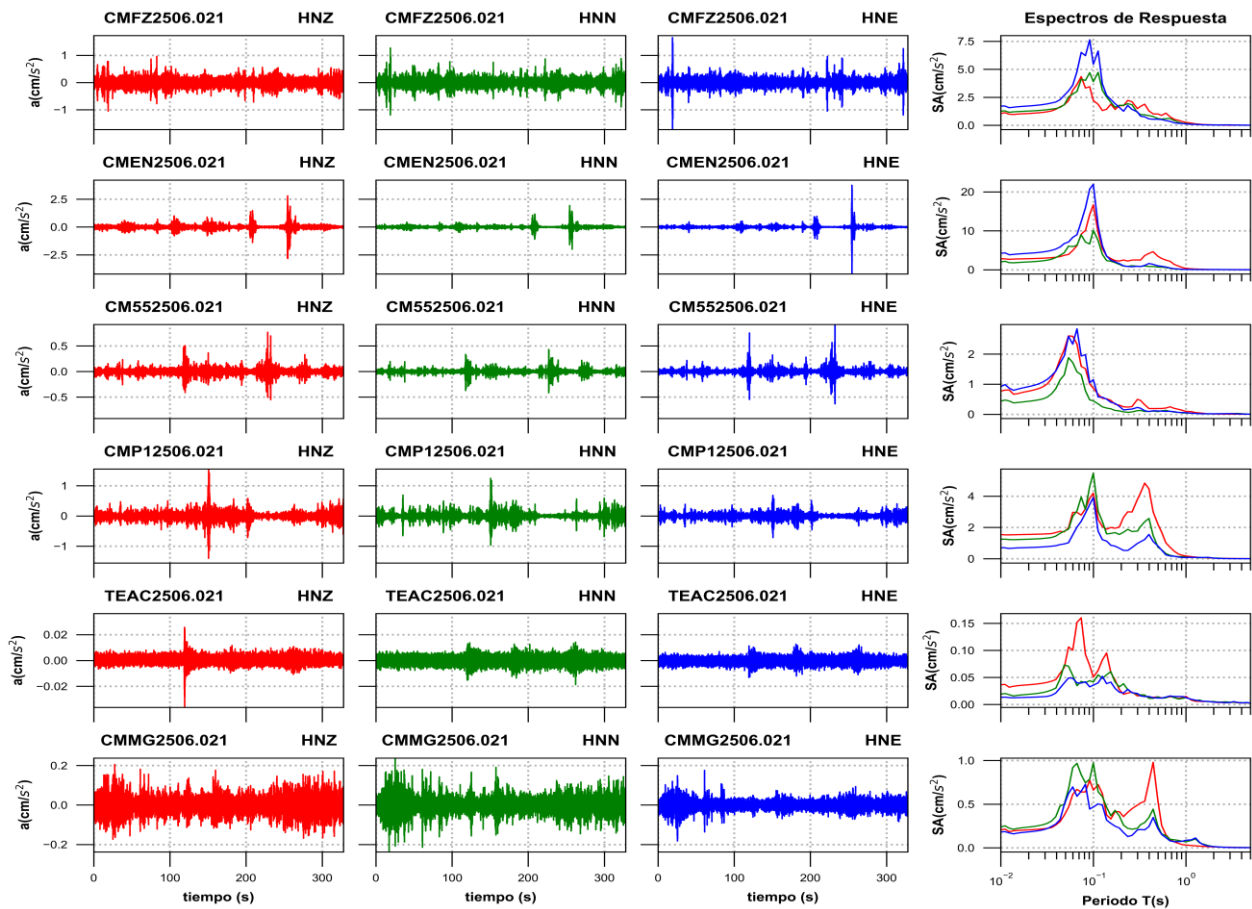
Figura 3c. Acelerogramas registrados y espectros de respuesta estimados para los registros obtenidos durante el sismo del 02 de junio de 2025 (M4.9)
