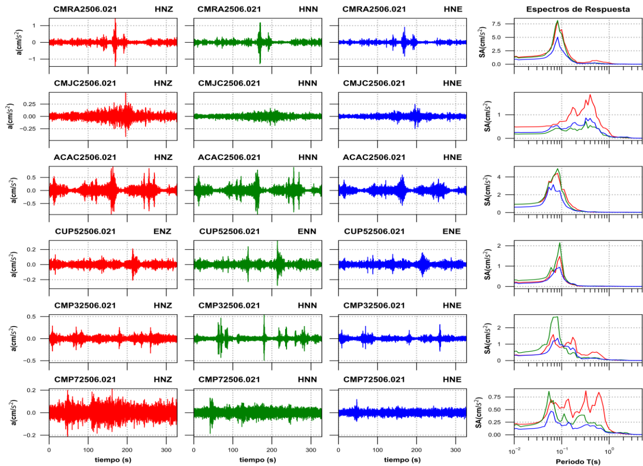
Figura 3e. Acelerogramas registrados y espectros de respuesta estimados para los registros obtenidos durante el sismo del 02 de junio de 2025 (M4.9)
