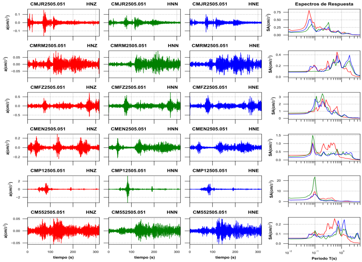
Figura 3c. Acelerogramas registrados y espectros de respuesta estimados para los registros obtenidos durante el sismo del 05 de mayo de 2025 (M5.7)
