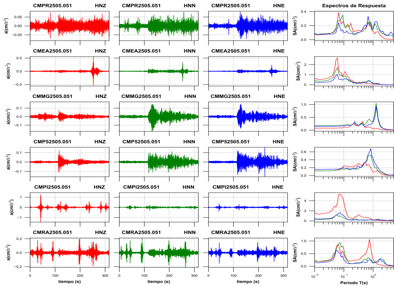
Figura 3d. Acelerogramas registrados y espectros de respuesta estimados para los registros obtenidos durante el sismo del 05 de mayo de 2025 (M5.7)
