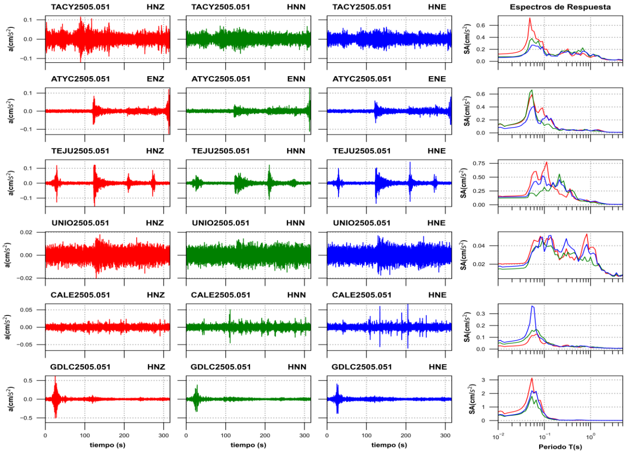
Figura 3g. Acelerogramas registrados y espectros de respuesta estimados para los registros obtenidos durante el sismo del 05 de mayo de 2025 (M5.7)
