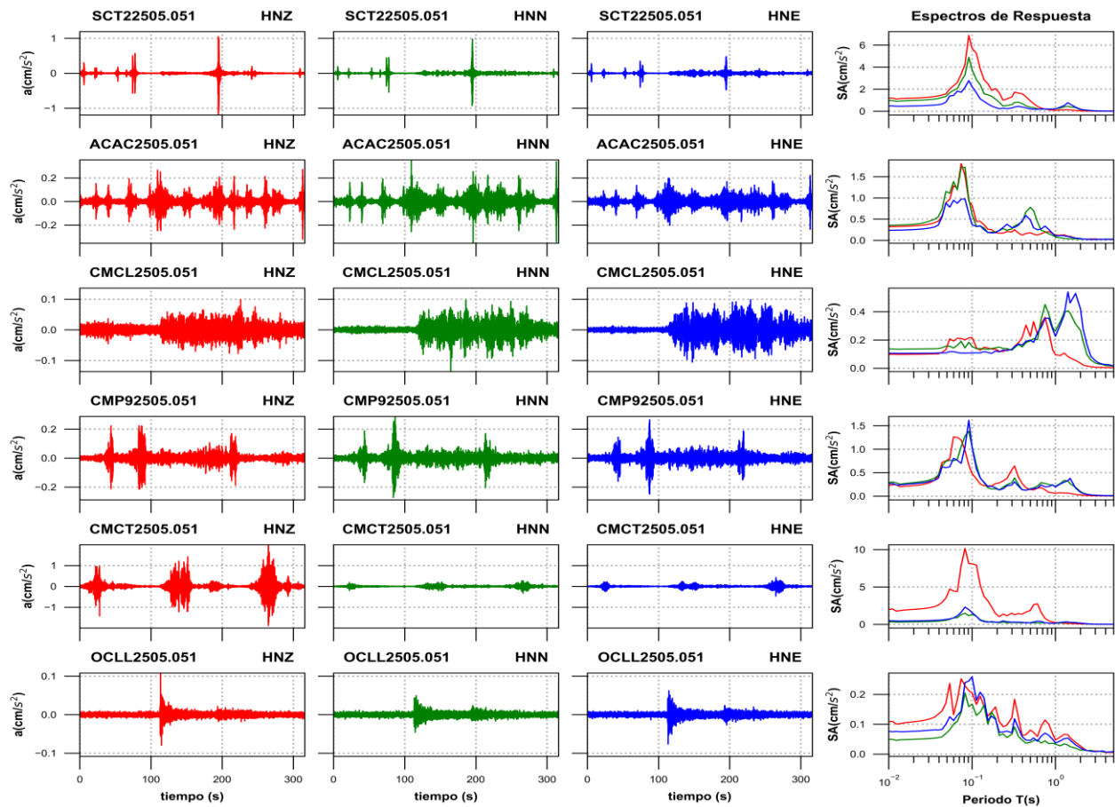
Figura 3f. Acelerogramas registrados y espectros de respuesta estimados para los registros obtenidos durante el sismo del 05 de mayo de 2025 (M5.7)
