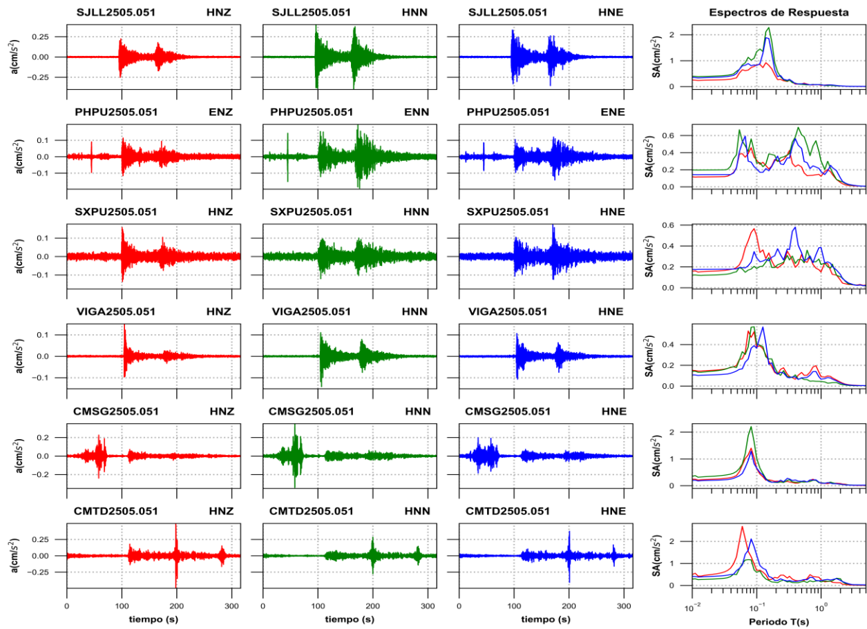
Figura 3b. Acelerogramas registrados y espectros de respuesta estimados para los registros obtenidos durante el sismo del 05 de mayo de 2025 (M5.7)
