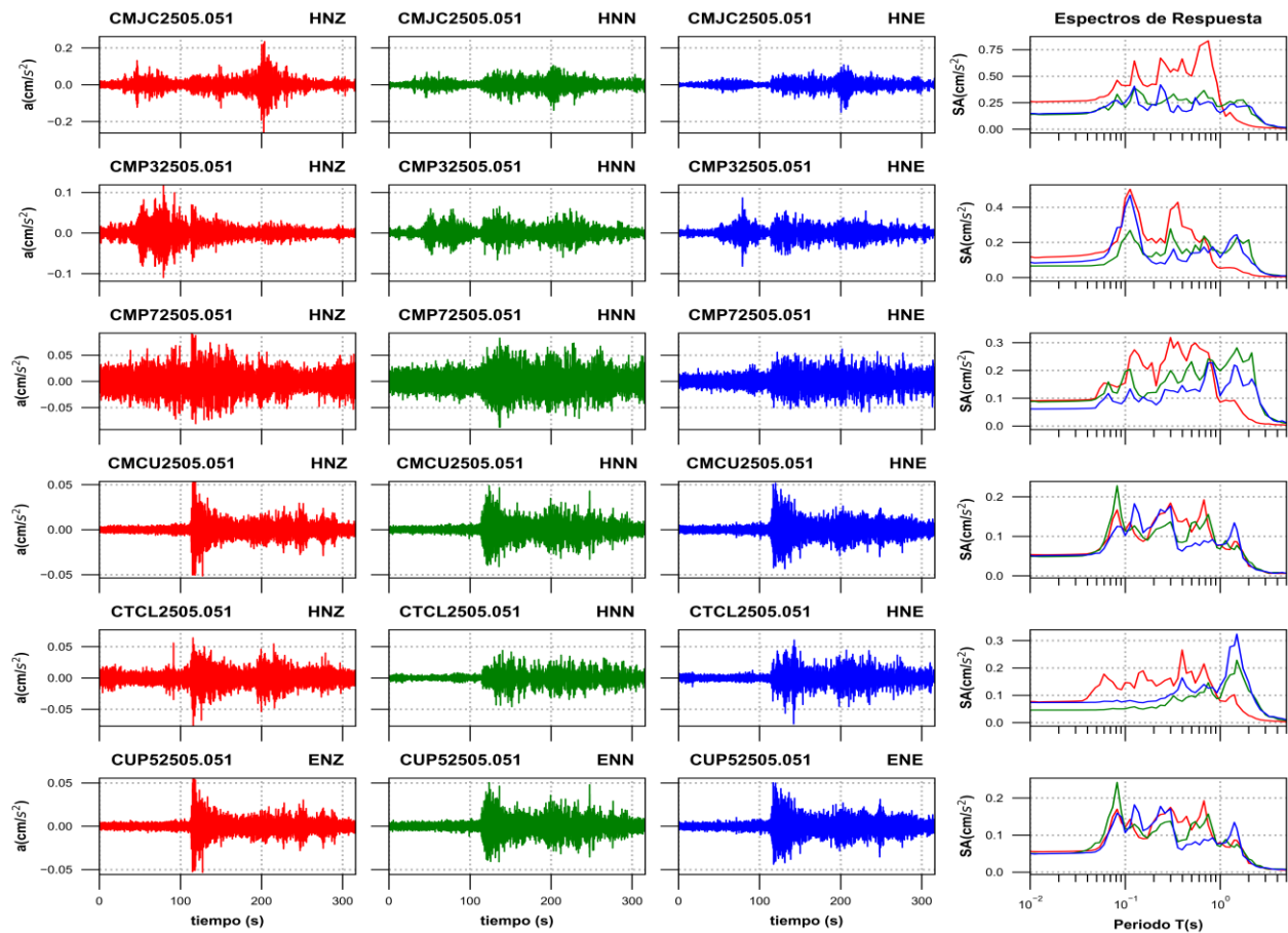
Figura 3e. Acelerogramas registrados y espectros de respuesta estimados para los registros obtenidos durante el sismo del 05 de mayo de 2025 (M5.7)
