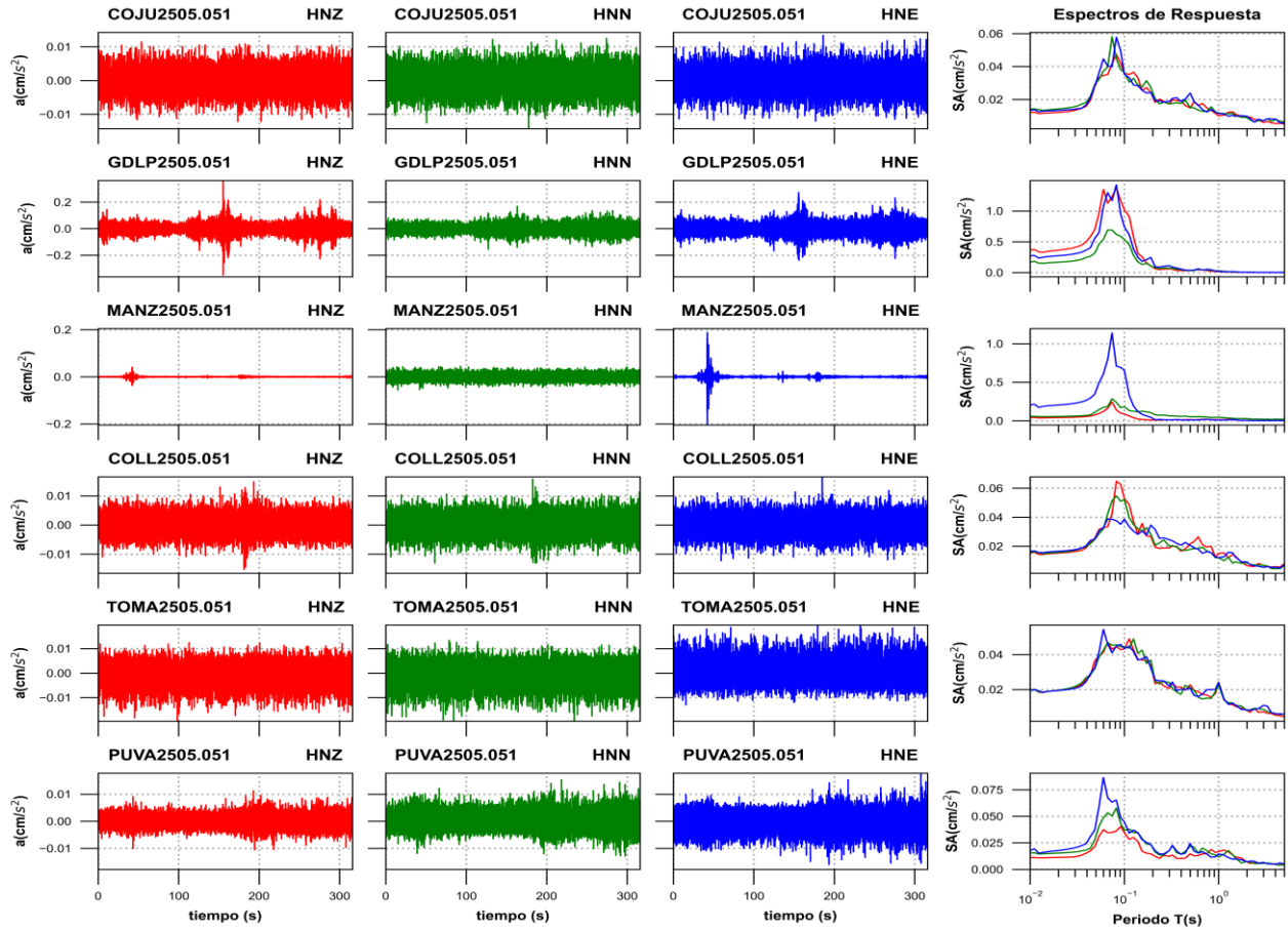
Figura 3h. Acelerogramas registrados y espectros de respuesta estimados para los registros obtenidos durante el sismo del 05 de mayo de 2025 (M5.7)
