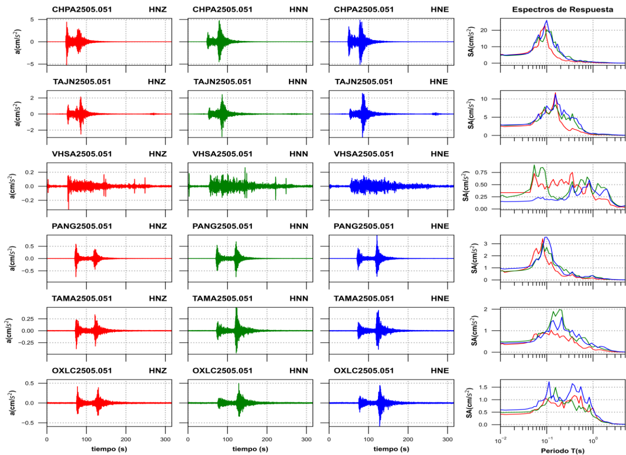
Figura 3a. Acelerogramas registrados y espectros de respuesta estimados para los registros obtenidos durante el sismo del 05 de mayo de 2025 (M5.7)
