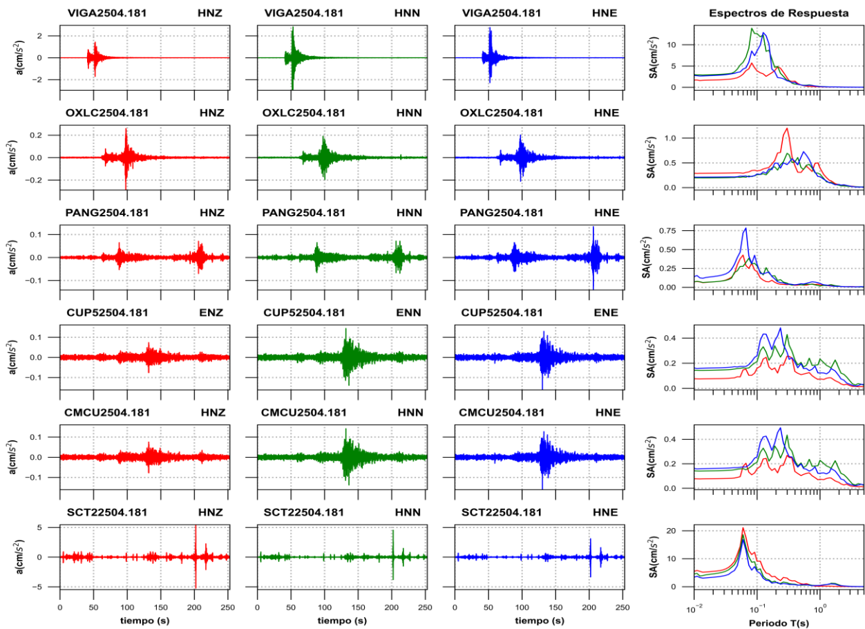
Figura 3a. Acelerogramas registrados y espectros de respuesta estimados para los registros obtenidos durante el sismo del 18 de abril de 2025 (M4.9)
