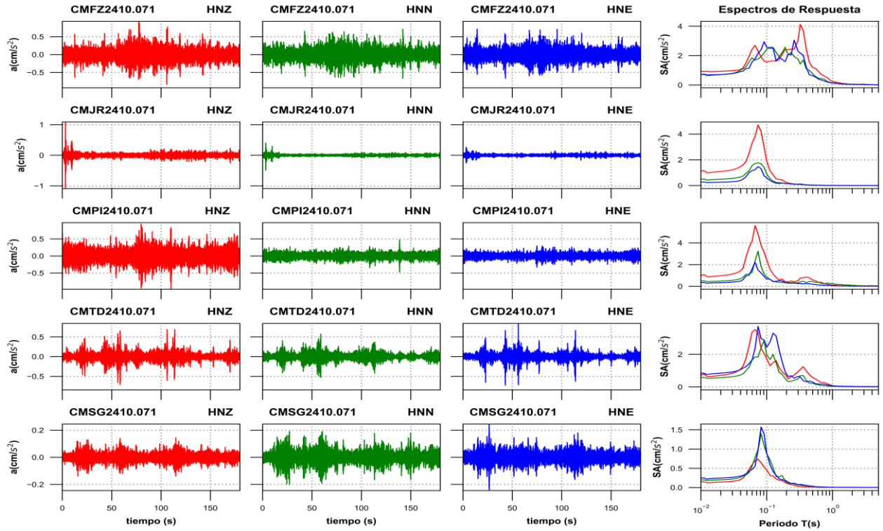
Figura 3f. Acelerogramas registrados y espectros de respuesta estimados para los registros obtenidos durante el sismo del 07 de octubre de 2024 (M2.0)
