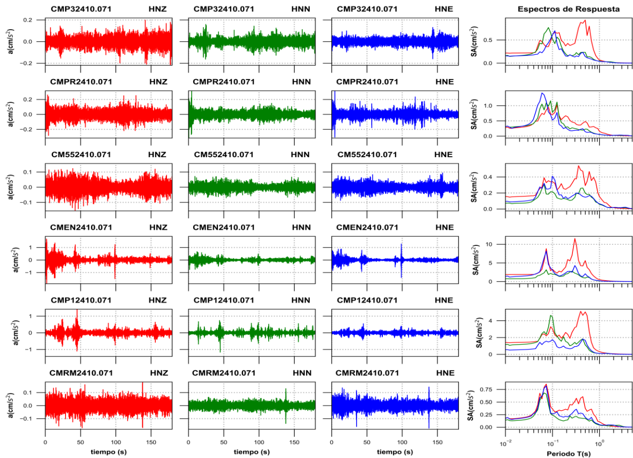
Figura 3e. Acelerogramas registrados y espectros de respuesta estimados para los registros obtenidos durante el sismo del 07 de octubre de 2024 (M2.0)
