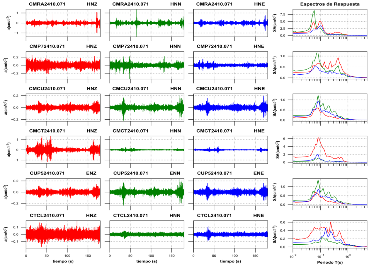
Figura 3c. Acelerogramas registrados y espectros de respuesta estimados para los registros obtenidos durante el sismo del 07 de octubre de 2024 (M2.0)
