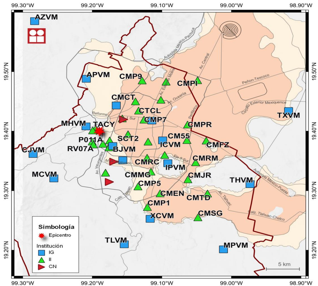
Figura 1. Epicentro del sismo del 07 de octubre de 2024 (M2.0) y estaciones sísmicas empleadas en la elaboración del mapa preliminar de PGA. Las estaciones pertenecientes a la Red Acelerográfica del Instituto de Ingeniería de la UNAM (RAII-UNAM) son operadas por la Unidad de Instrumentación Sísmica. Las estaciones IG y CN mostradas son operadas por el Servicio Sismológico Nacional y el Centro Nacional de Prevención de Desastres, respectivamente.
