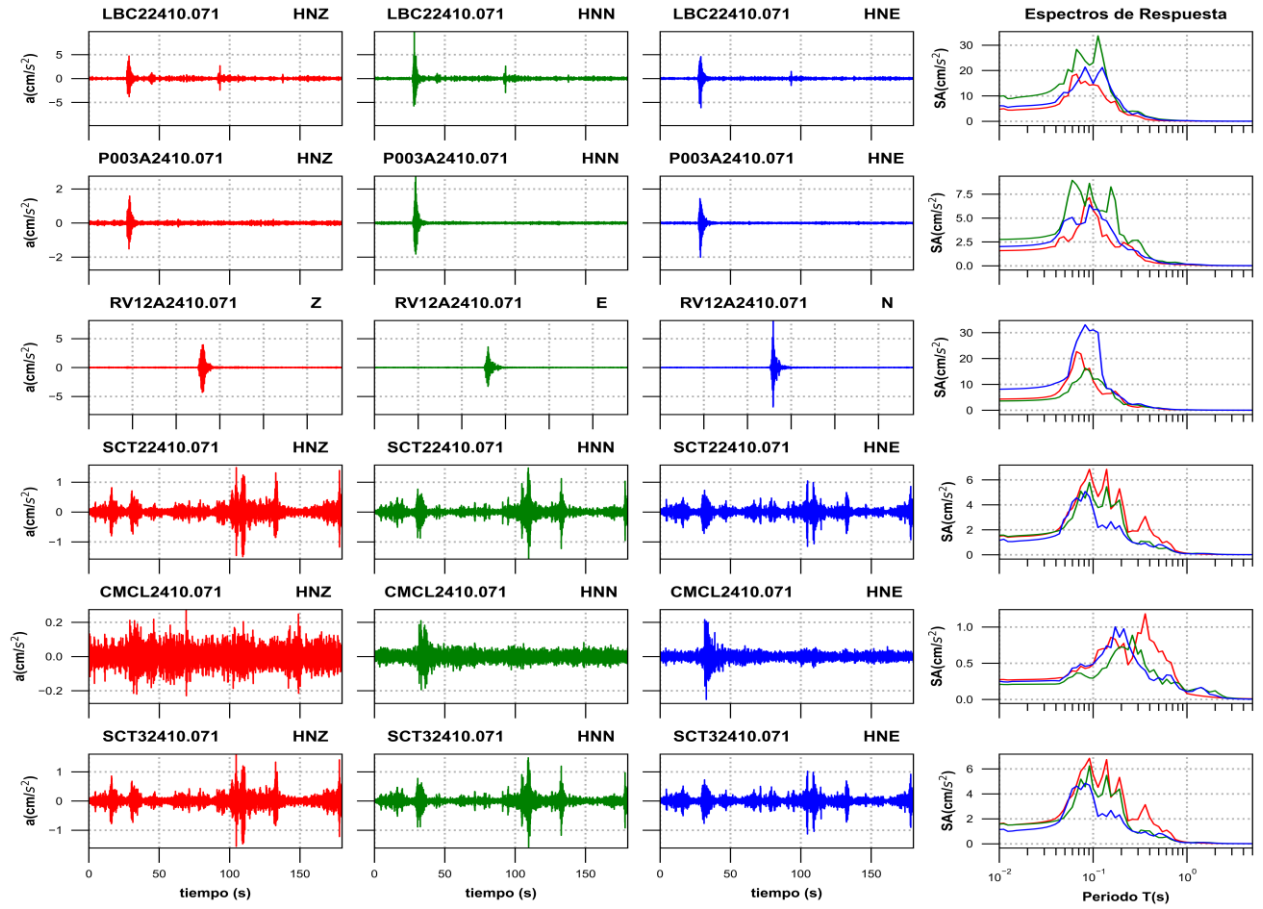
Figura 3b. Acelerogramas registrados y espectros de respuesta estimados para los registros obtenidos durante el sismo del 07 de octubre de 2024 (M2.0)
