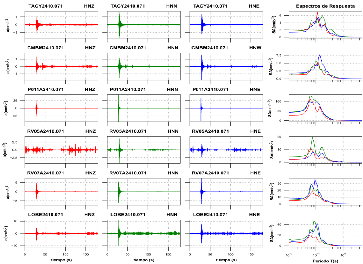
Figura 3a. Acelerogramas registrados y espectros de respuesta estimados para los registros obtenidos durante el sismo del 07 de octubre de 2024 (M2.0)
