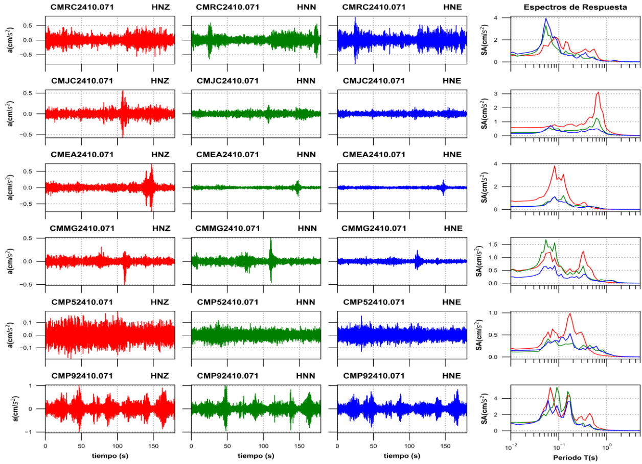
Figura 3d. Acelerogramas registrados y espectros de respuesta estimados para los registros obtenidos durante el sismo del 07 de octubre de 2024 (M2.0)
