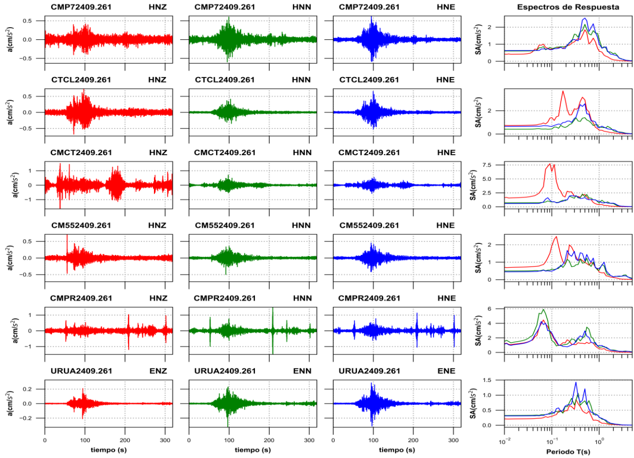
Figura 3d. Acelerogramas registrados y espectros de respuesta estimados para los registros obtenidos durante el sismo del 26 de septiembre de 2024 (M5.2)
