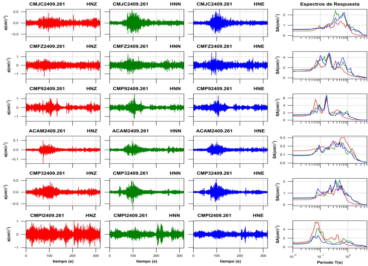
Figura 3e. Acelerogramas registrados y espectros de respuesta estimados para los registros obtenidos durante el sismo del 26 de septiembre de 2024 (M5.2)
