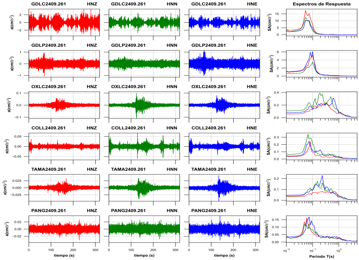
Figura 3g. Acelerogramas registrados y espectros de respuesta estimados para los registros obtenidos durante el sismo del 26 de septiembre de 2024 (M5.2)
