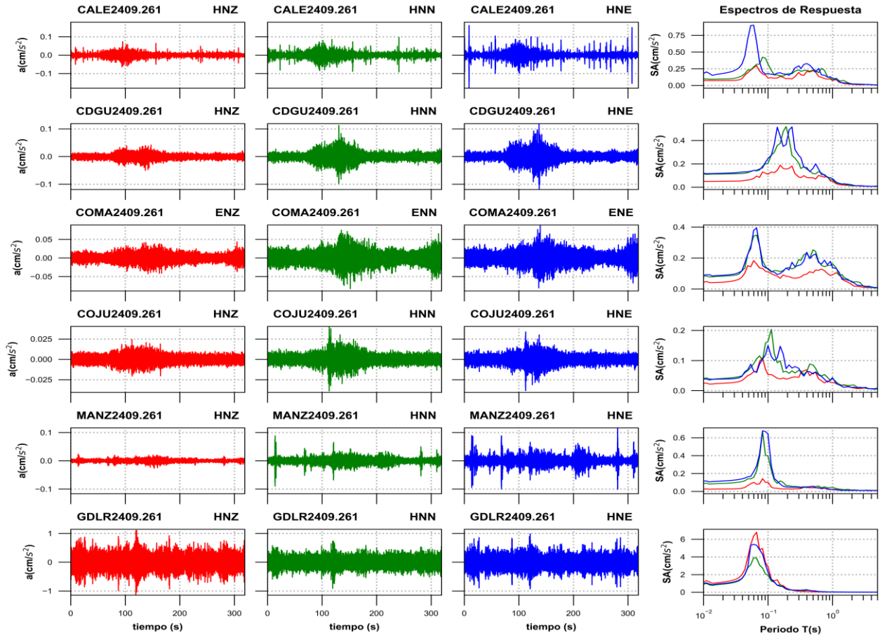
Figura 3f. Acelerogramas registrados y espectros de respuesta estimados para los registros obtenidos durante el sismo del 26 de septiembre de 2024 (M5.2)
