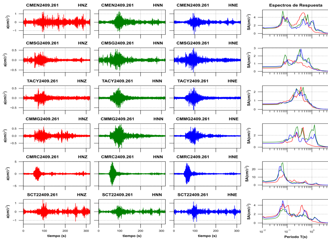
Figura 3b. Acelerogramas registrados y espectros de respuesta estimados para los registros obtenidos durante el sismo del 26 de septiembre de 2024 (M5.2)
