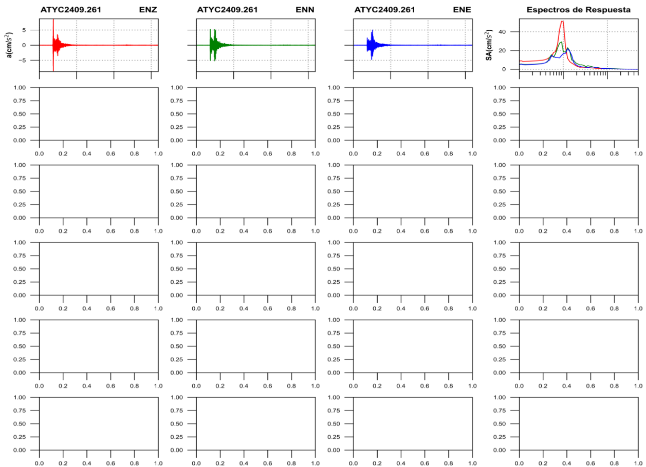
Figura 3a. Acelerogramas registrados y espectros de respuesta estimados para los registros obtenidos durante el sismo del 26 de septiembre de 2024 (M5.2)
