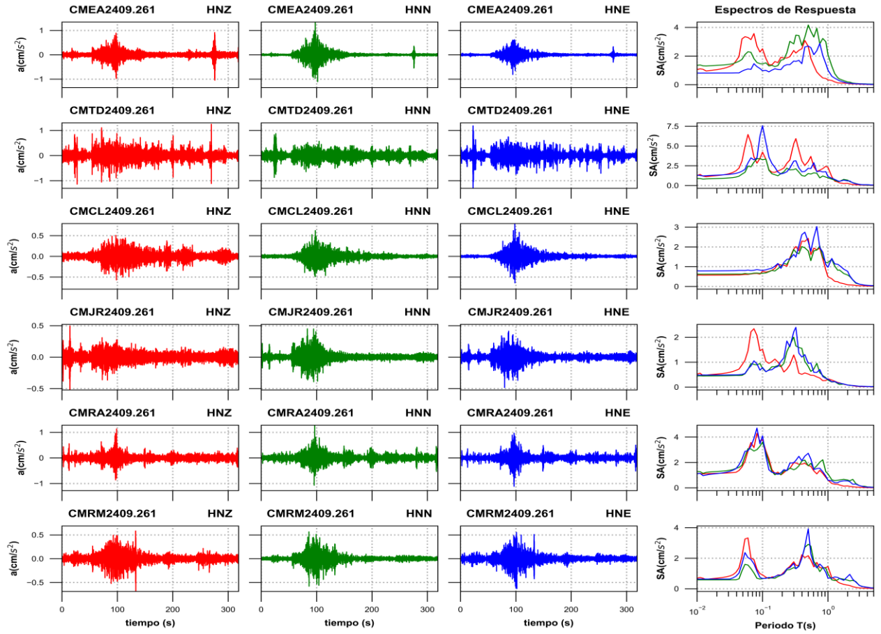
Figura 3c. Acelerogramas registrados y espectros de respuesta estimados para los registros obtenidos durante el sismo del 26 de septiembre de 2024 (M5.2)
