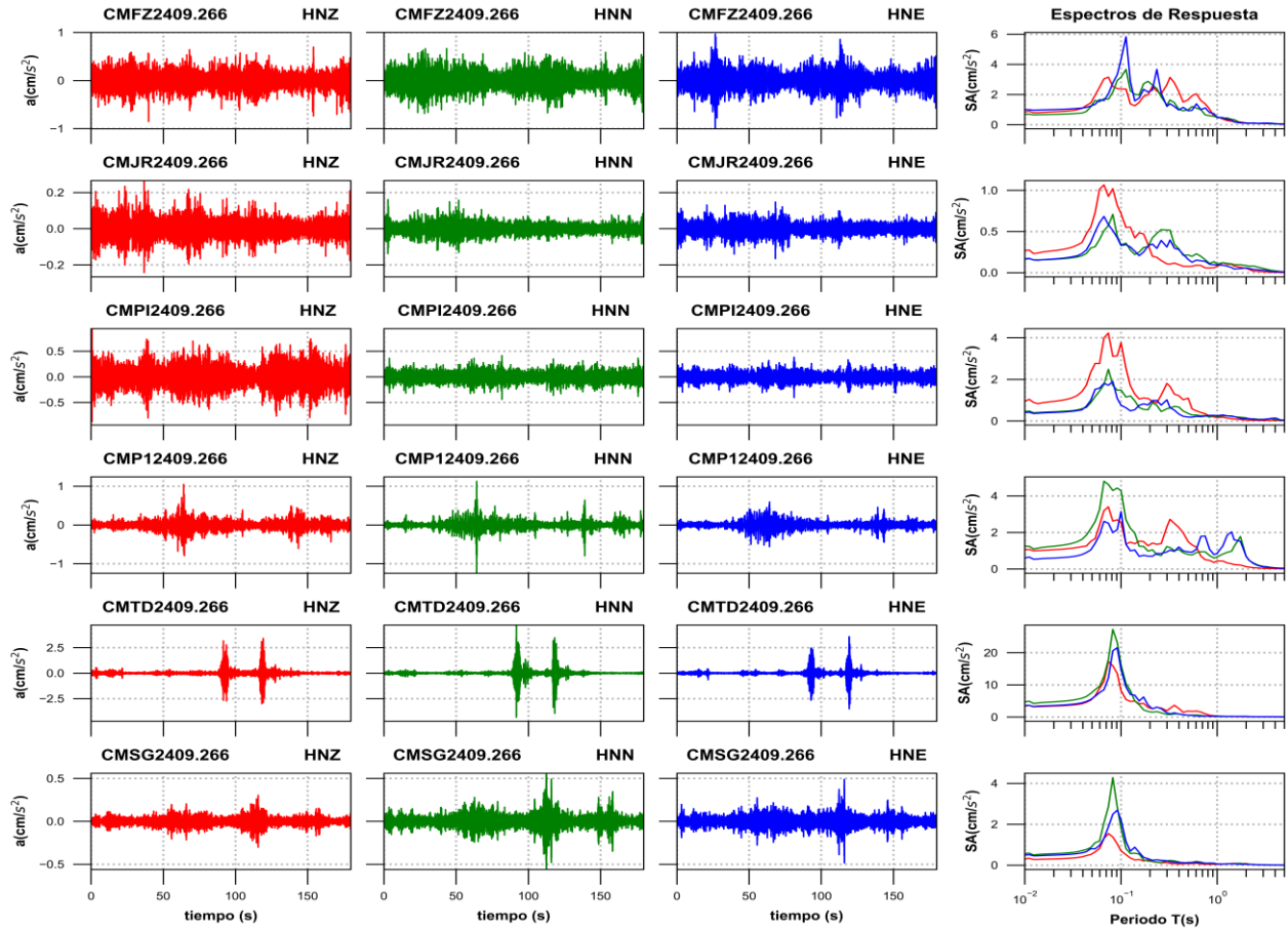
Figura 3e. Acelerogramas registrados y espectros de respuesta estimados para los registros obtenidos durante el sismo del 26 de septiembre de 2024 (M2.4)
