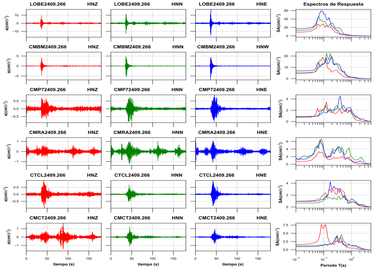
Figura 3b. Acelerogramas registrados y espectros de respuesta estimados para los registros obtenidos durante el sismo del 26 de septiembre de 2024 (M2.4)
