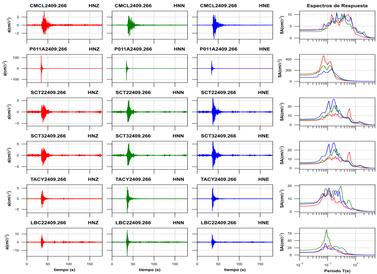
Figura 3a. Acelerogramas registrados y espectros de respuesta estimados para los registros obtenidos durante el sismo del 26 de septiembre de 2024 (M2.4)
