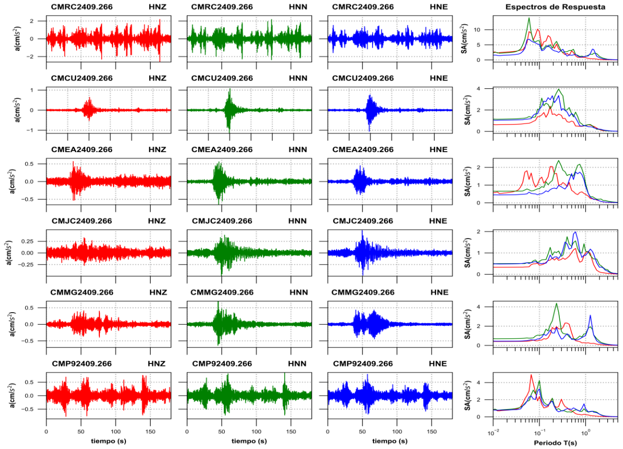
Figura 3c. Acelerogramas registrados y espectros de respuesta estimados para los registros obtenidos durante el sismo del 26 de septiembre de 2024 (M2.4)
