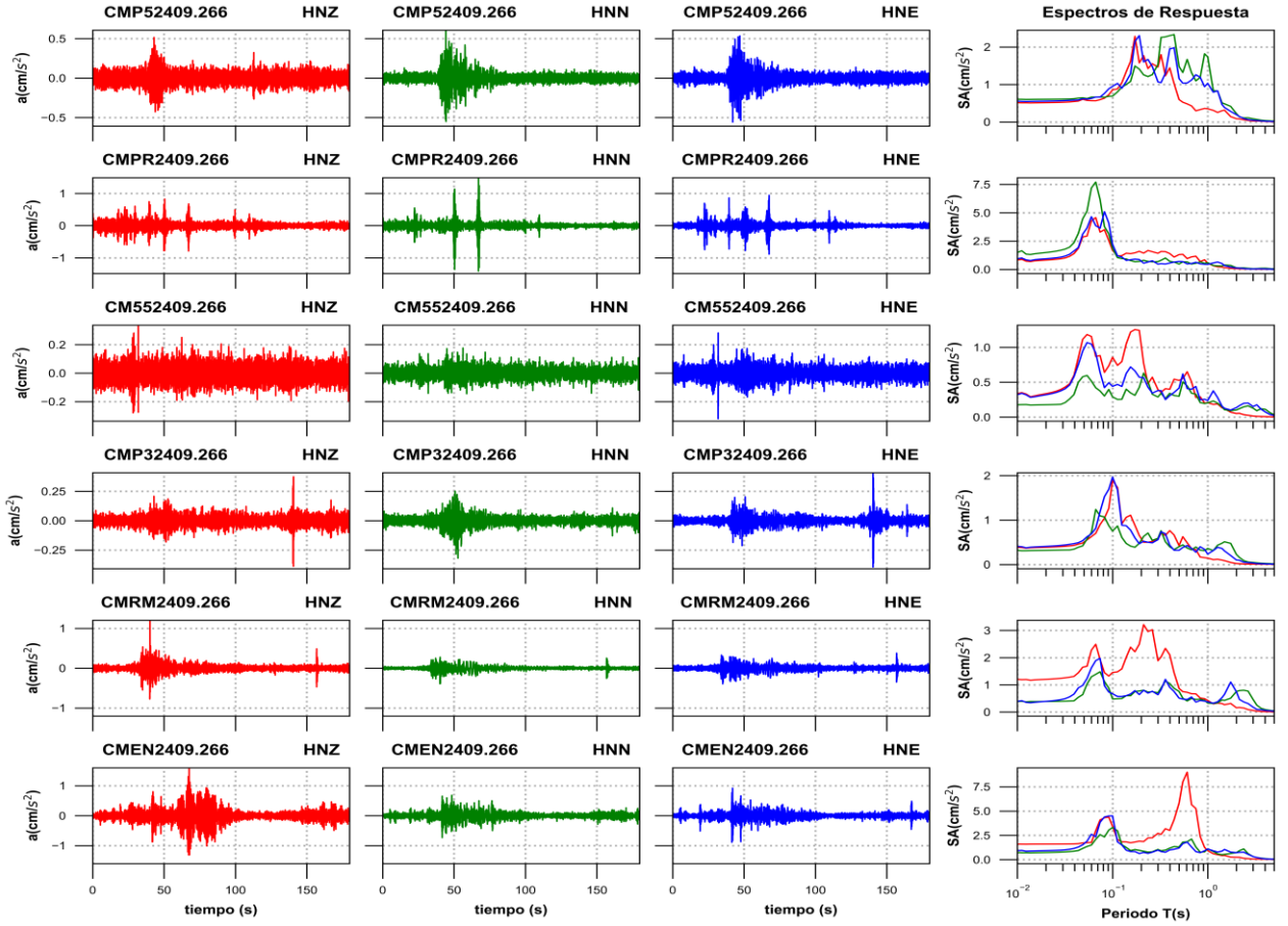
Figura 3d. Acelerogramas registrados y espectros de respuesta estimados para los registros obtenidos durante el sismo del 26 de septiembre de 2024 (M2.4)
