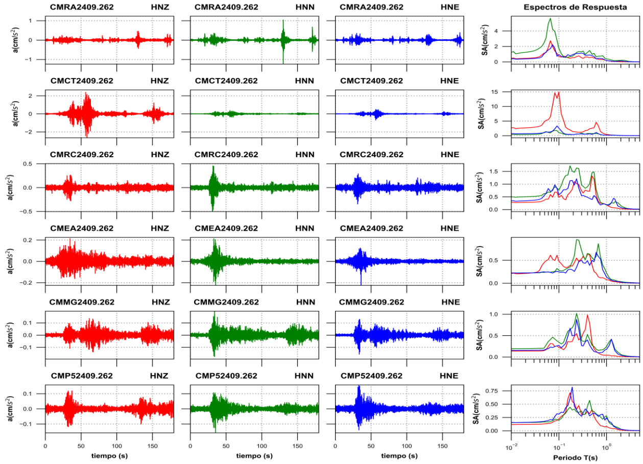
Figura 3c. Acelerogramas registrados y espectros de respuesta estimados para los registros obtenidos durante el sismo del 26 de septiembre de 2024 (M2.0)
