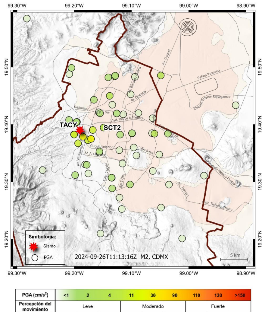
Figura 2. Mapa de Aceleraciones Máximas registradas ( PGA_{rms} )
