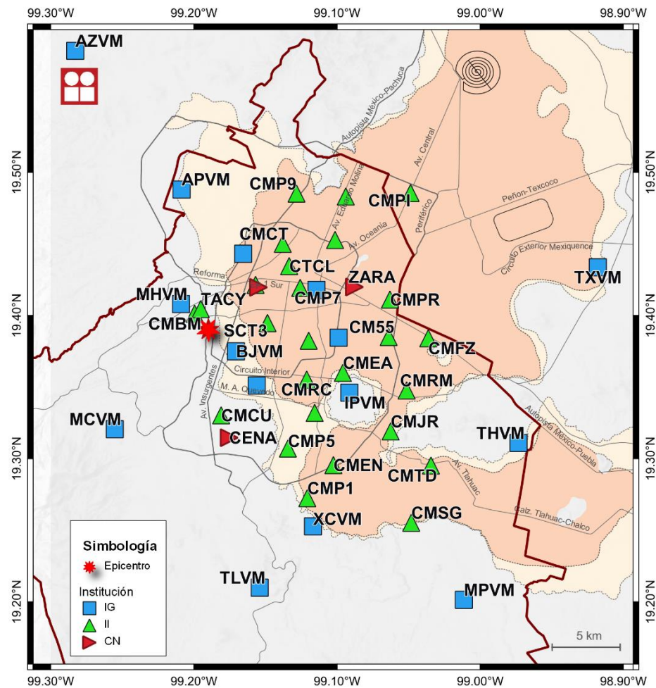
Figura 1. Epicentro del sismo del 26 de septiembre de 2024 (M2.0) y estaciones sísmicas empleadas en la elaboración del mapa preliminar de PGA. Las estaciones pertenecientes a la Red Acelerográfica del Instituto de Ingeniería de la UNAM (RAII-UNAM) son operadas por la Unidad de Instrumentación Sísmica. Las estaciones IG y CN mostradas son operadas por el Servicio Sismológico Nacional y el Centro Nacional de Prevención de Desastres, respectivamente.
