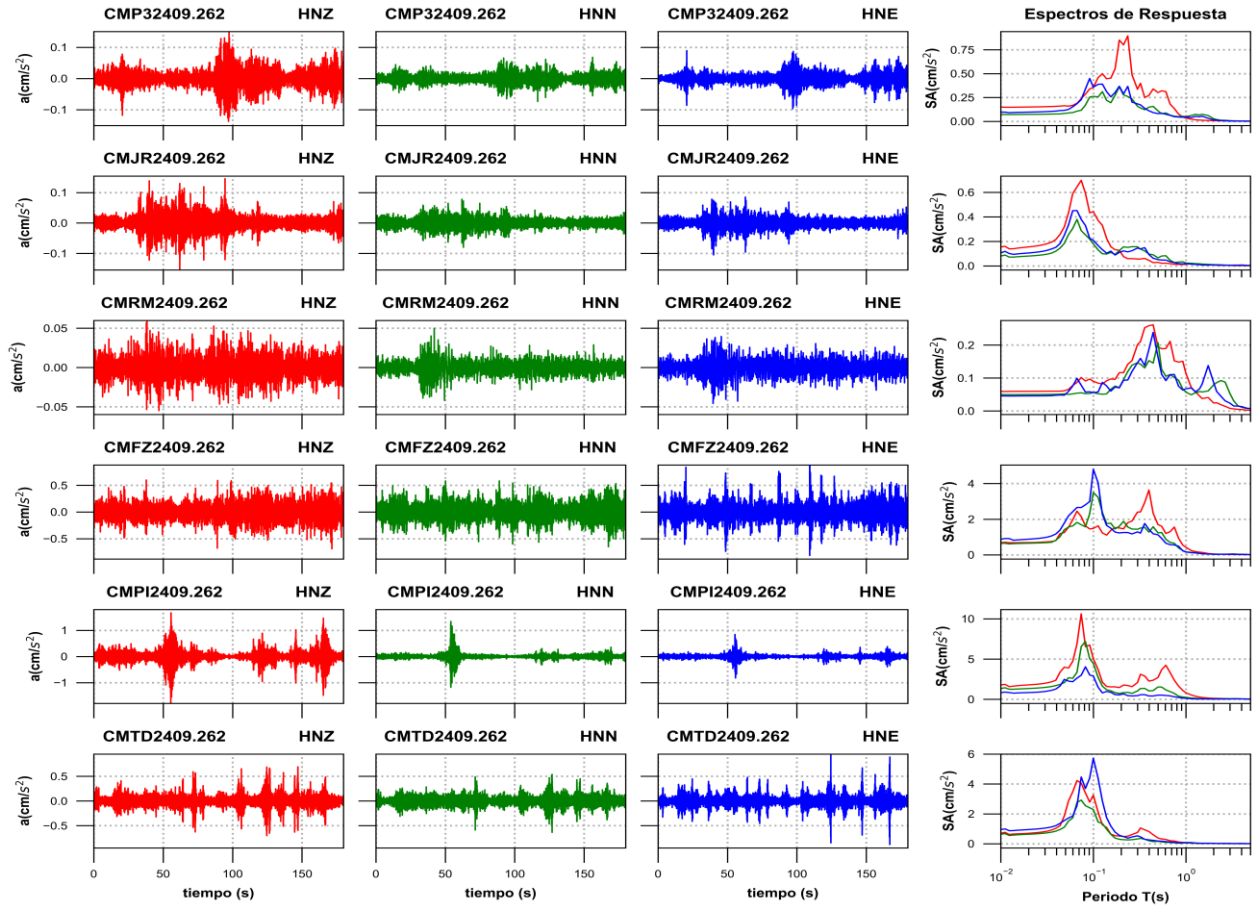
Figura 3e. Acelerogramas registrados y espectros de respuesta estimados para los registros obtenidos durante el sismo del 26 de septiembre de 2024 (M2.0)
