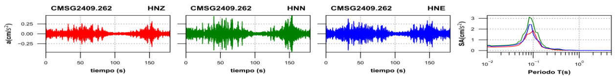
Figura 3f. Acelerogramas registrados y espectros de respuesta estimados para los registros obtenidos durante el sismo del 26 de septiembre de 2024 (M2.0)
