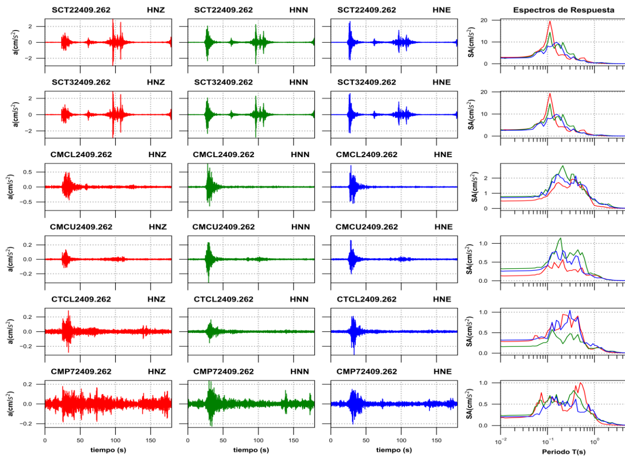
Figura 3b. Acelerogramas registrados y espectros de respuesta estimados para los registros obtenidos durante el sismo del 26 de septiembre de 2024 (M2.0)
