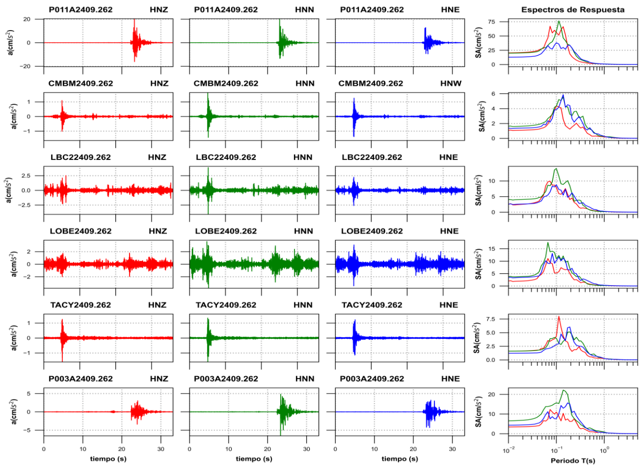
Figura 3a. Acelerogramas registrados y espectros de respuesta estimados para los registros obtenidos durante el sismo del 26 de septiembre de 2024 (M2.0)
