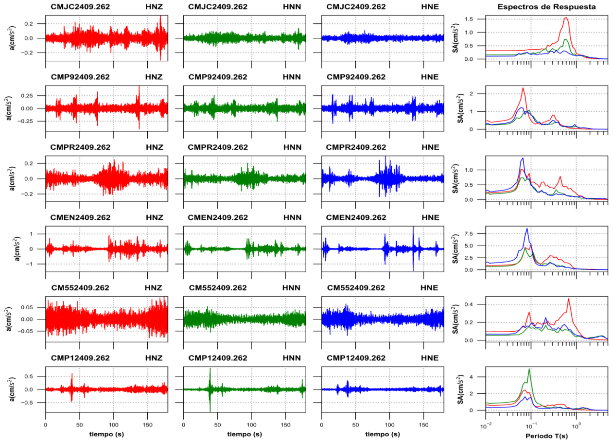
Figura 3d. Acelerogramas registrados y espectros de respuesta estimados para los registros obtenidos durante el sismo del 26 de septiembre de 2024 (M2.0)
