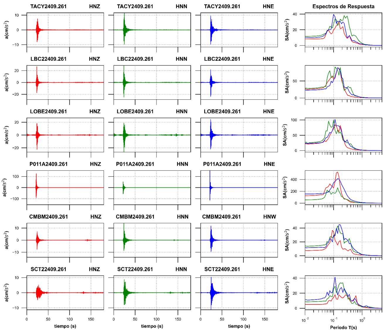
Figura 3a. Acelerogramas registrados y espectros de respuesta estimados para los registros obtenidos durante el sismo del 26 de septiembre de 2024 (M2.9)
