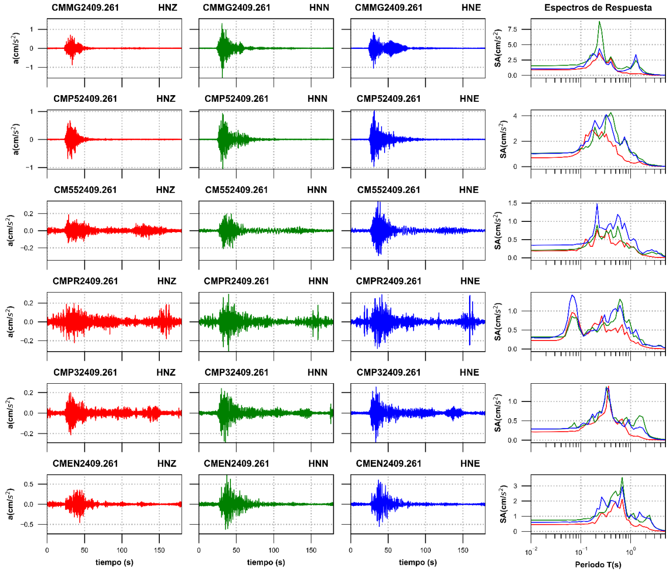
Figura 3d. Acelerogramas registrados y espectros de respuesta estimados para los registros obtenidos durante el sismo del 26 de septiembre de 2024 (M2.9)
