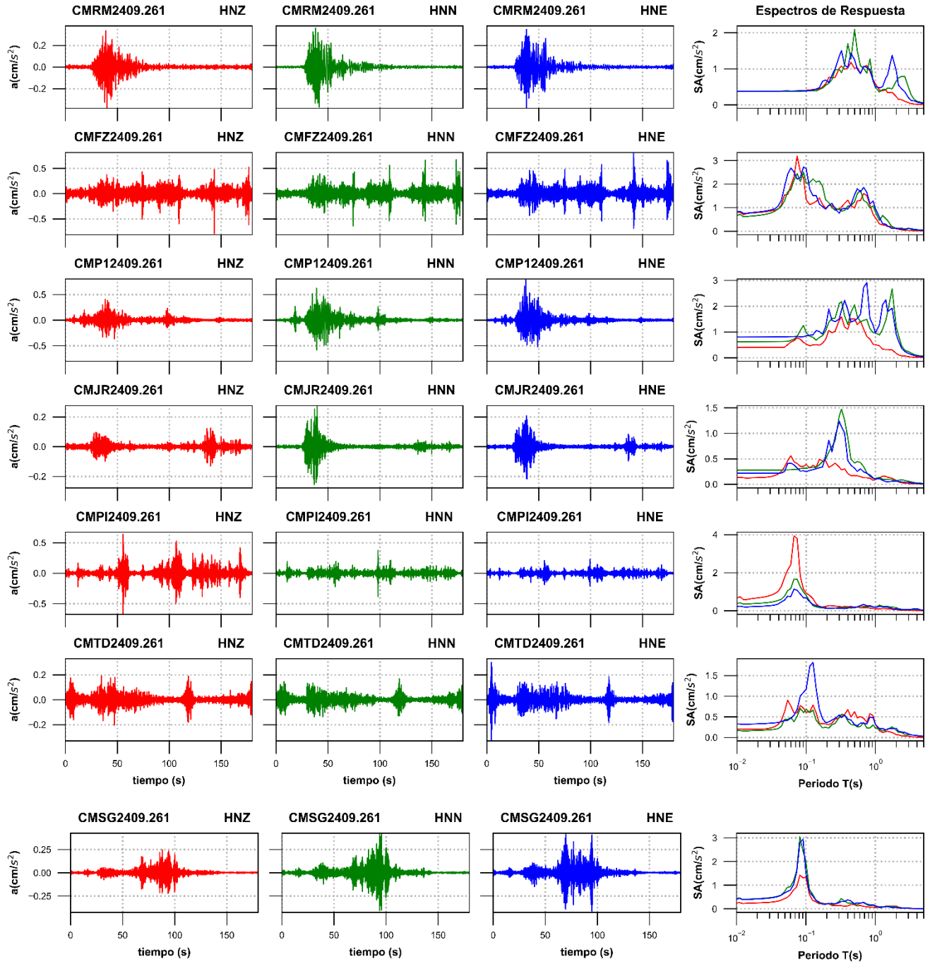
Figura 3e. Acelerogramas registrados y espectros de respuesta estimados para los registros obtenidos durante el sismo del 26 de septiembre de 2024 (M2.9)
