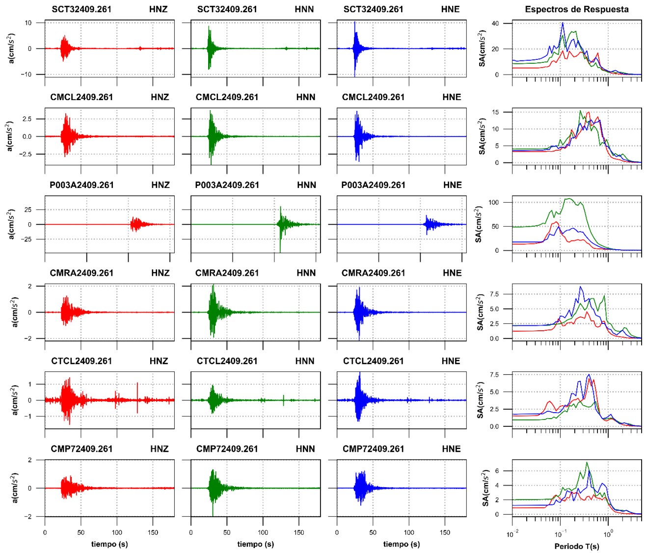
Figura 3b. Acelerogramas registrados y espectros de respuesta estimados para los registros obtenidos durante el sismo del 26 de septiembre de 2024 (M2.9)
