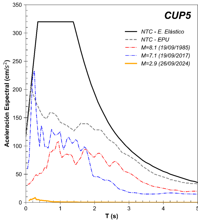
Figura 4. Comparación del espectro de respuesta (ER) del sismo registrado en la estación CUP5 con el espectro elástico de diseño (EDS) y de peligro uniforme (EPU) obtenidos del SASID. La línea discontinua de color rojo y azul corresponden a los ER de los sismos del 19 septiembre de 1985 y 2017, respectivamente. Todos los ER graficados corresponden a la media cuadrática de sus componentes horizontales.
