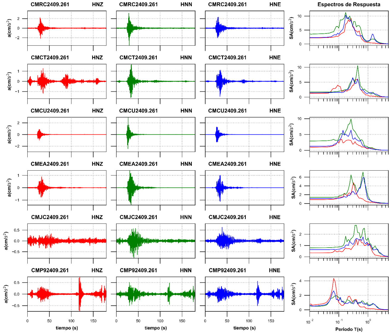
Figura 3c. Acelerogramas registrados y espectros de respuesta estimados para los registros obtenidos durante el sismo del 26 de septiembre de 2024 (M2.9)
