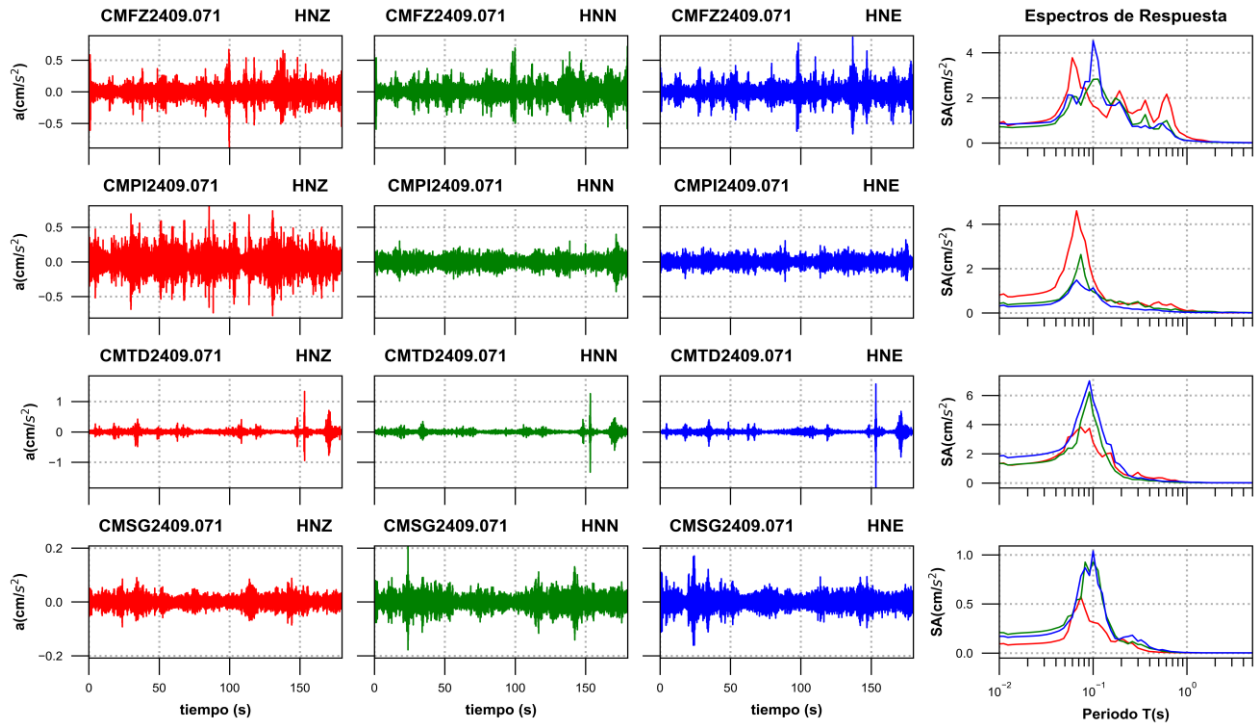
Figura 3e. Acelerogramas registrados y espectros de respuesta estimados para los registros obtenidos durante el sismo del 06 de septiembre de 2024 (M2.2)
