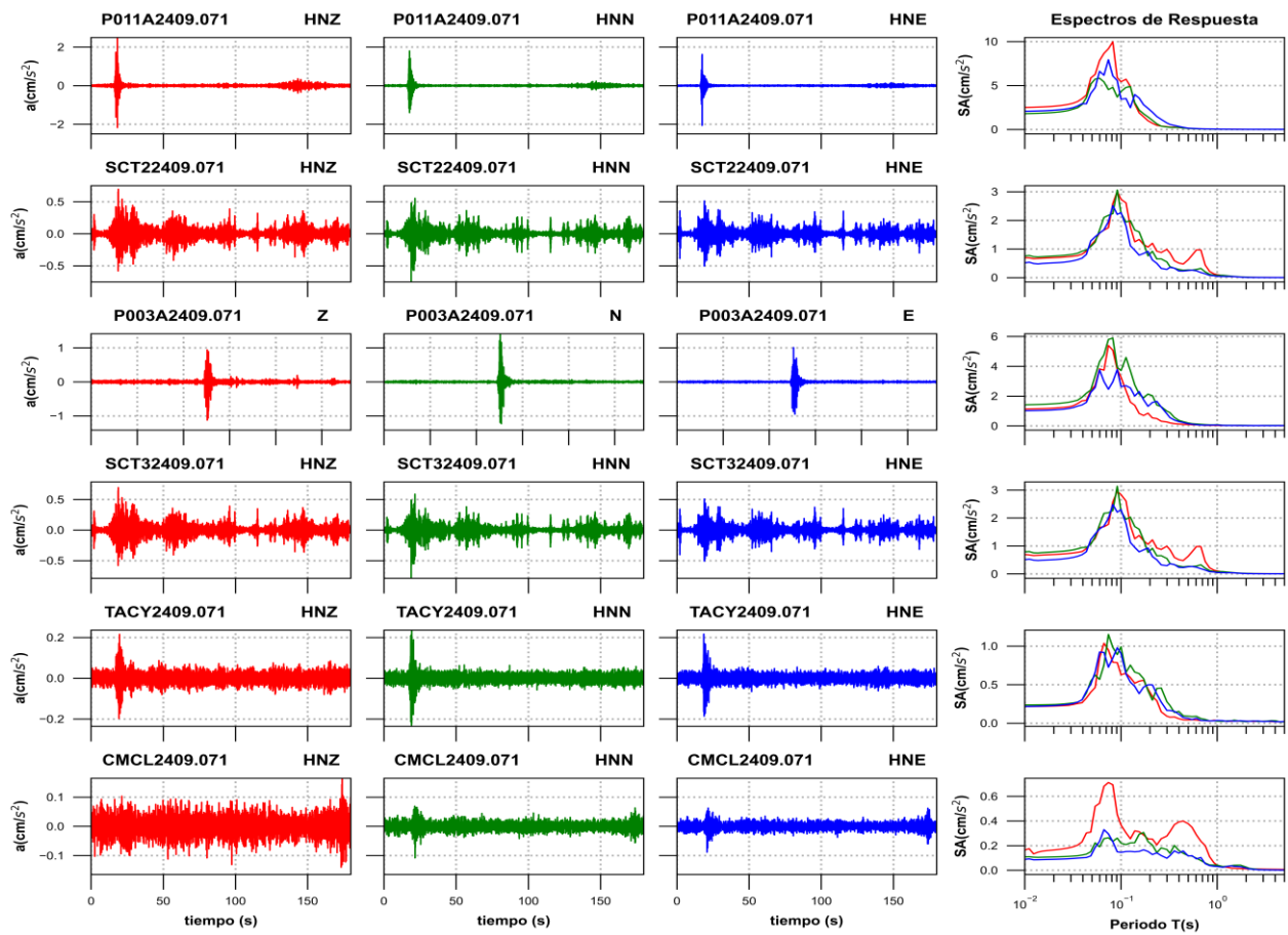
Figura 3a. Acelerogramas registrados y espectros de respuesta estimados para los registros obtenidos durante el sismo del 06 de septiembre de 2024 (M2.2)
