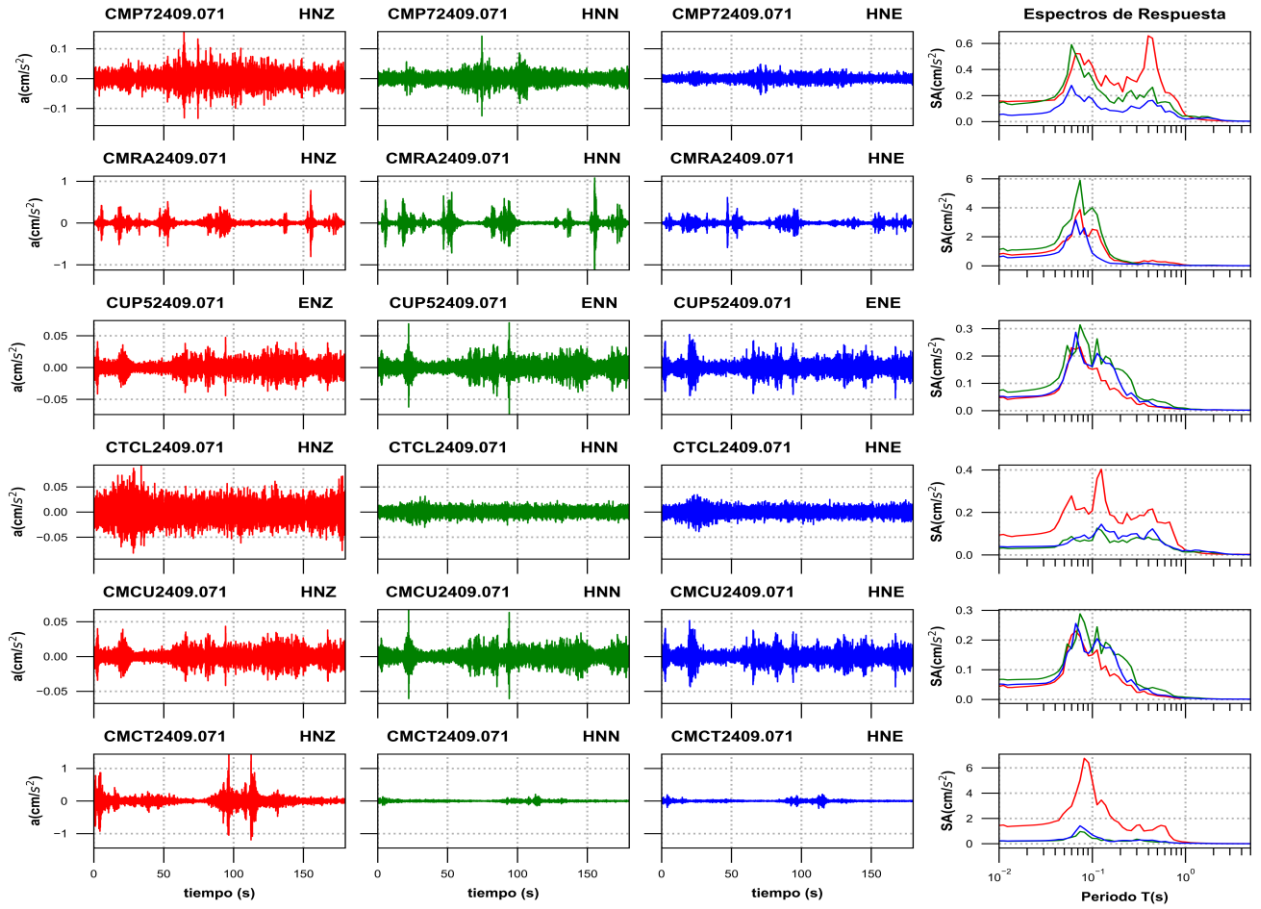
Figura 3b. Acelerogramas registrados y espectros de respuesta estimados para los registros obtenidos durante el sismo del 06 de septiembre de 2024 (M2.2)
