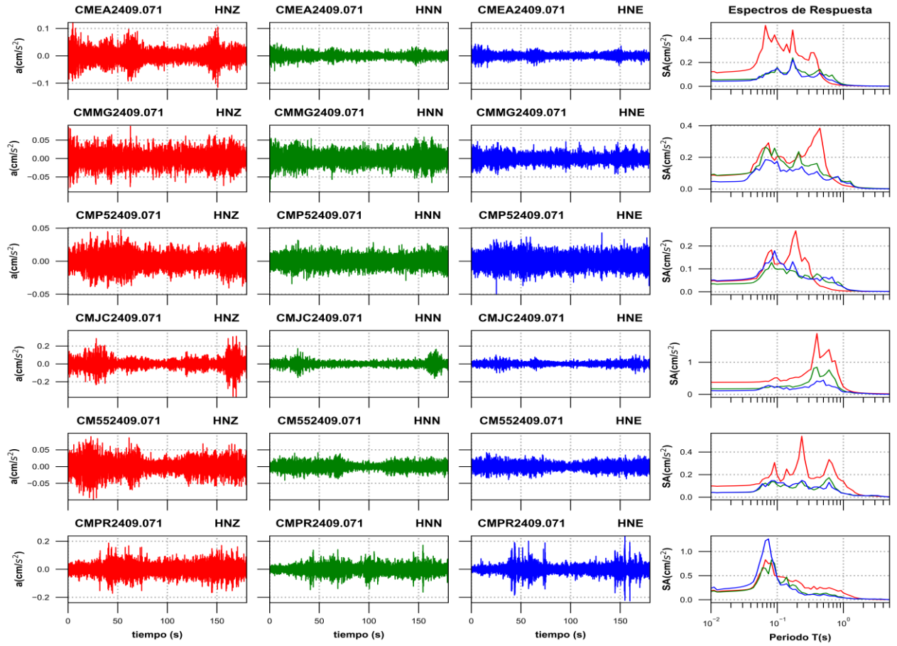
Figura 3c. Acelerogramas registrados y espectros de respuesta estimados para los registros obtenidos durante el sismo del 06 de septiembre de 2024 (M2.2)
