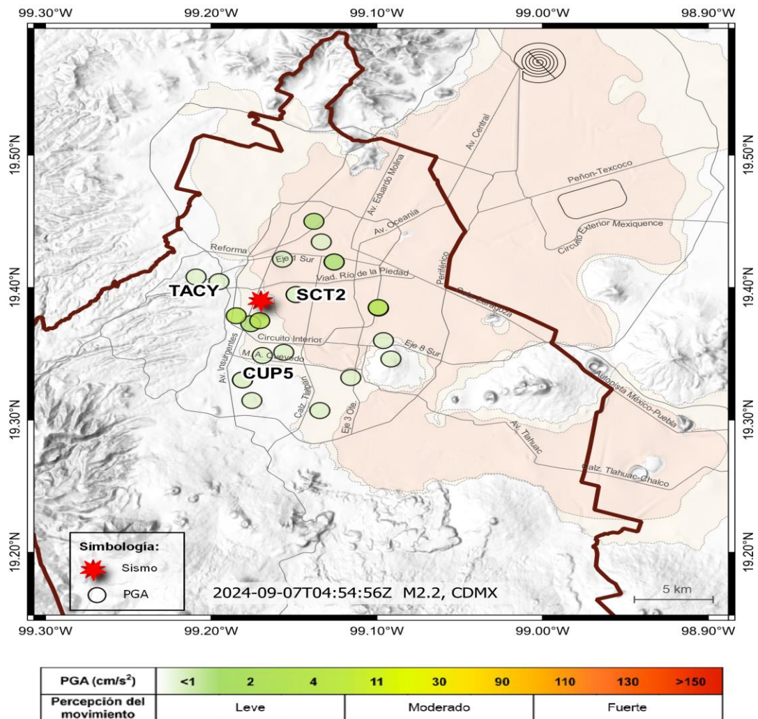
Figura 2. Mapa preliminar de Aceleración Máxima del Terreno ( PGA_{rms} ) en la Ciudad de México.
