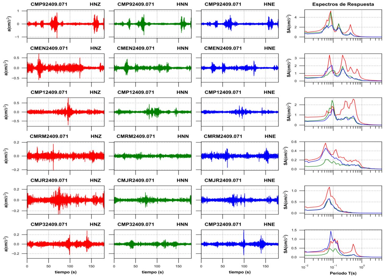
Figura 3d. Acelerogramas registrados y espectros de respuesta estimados para los registros obtenidos durante el sismo del 06 de septiembre de 2024 (M2.2)
