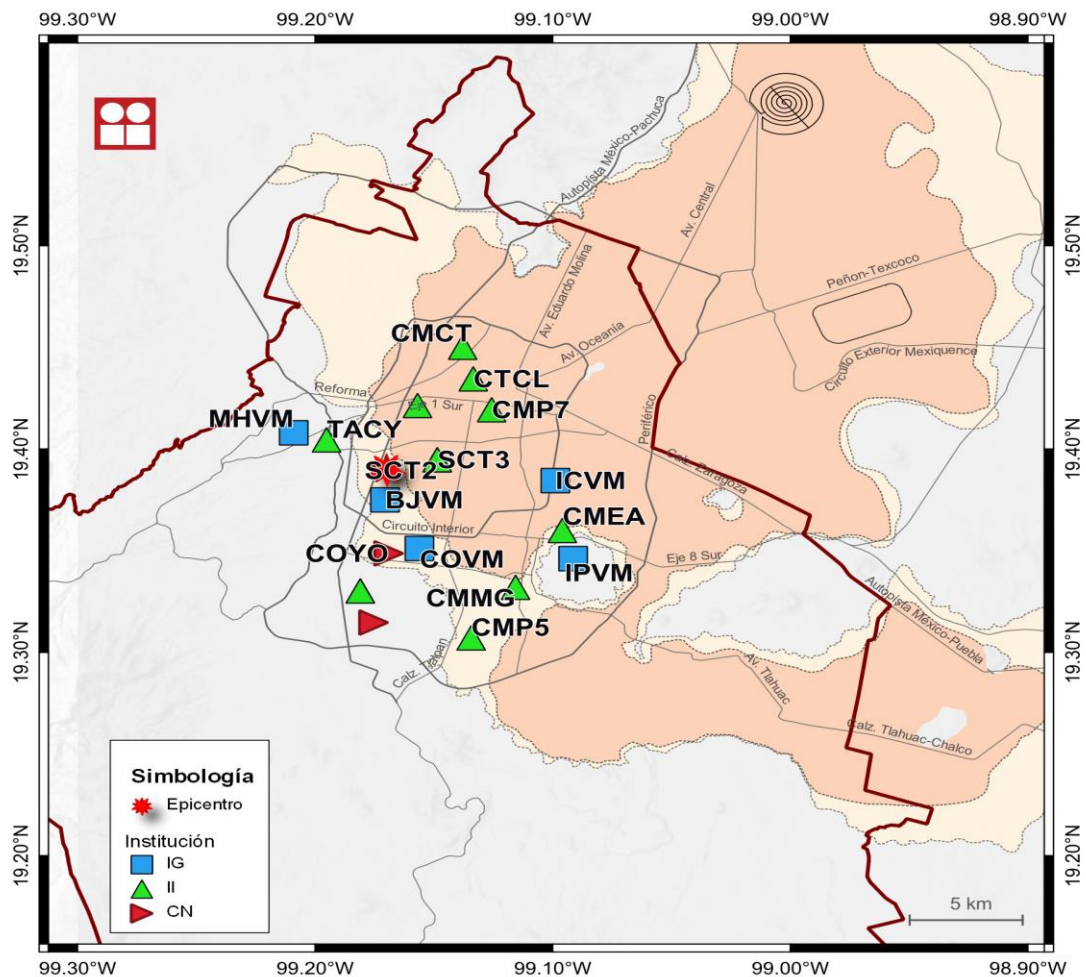
Figura 1. Epicentro del sismo del 06 de septiembre de 2024 (M2.2) y estaciones sísmicas empleadas en la elaboración del mapa preliminar de PGA. Las estaciones pertenecientes a la Red Acelerográfica del Instituto de Ingeniería de la UNAM (IIUNAM) son operadas por la Unidad de Instrumentación Sísmica. Las estaciones IG y CN mostradas son operadas por el Servicio Sismológico Nacional y el Centro Nacional de Prevención de Desastres, respectivamente.
