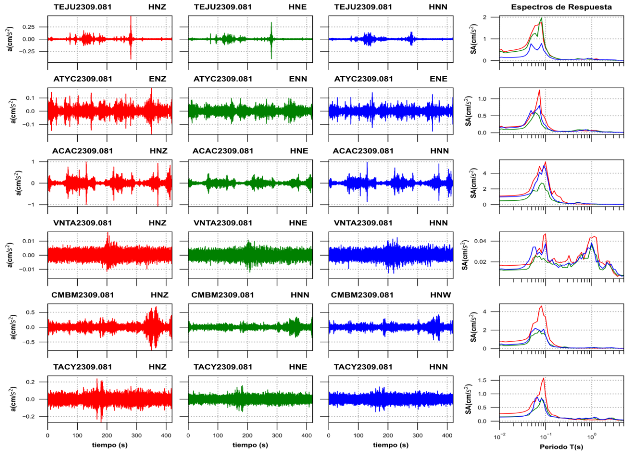
Figura 3b. Acelerogramas registrados y espectros de respuesta estimados para los registros obtenidos durante el sismo del 08 de septiembre de 2023 (M5.7)
