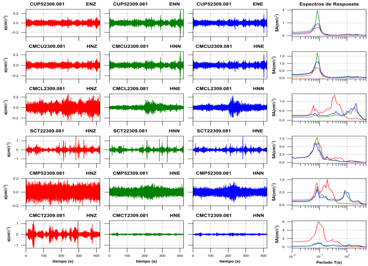
Figura 3c. Acelerogramas registrados y espectros de respuesta estimados para los registros obtenidos durante el sismo del 08 de septiembre de 2023 (M5.7)
