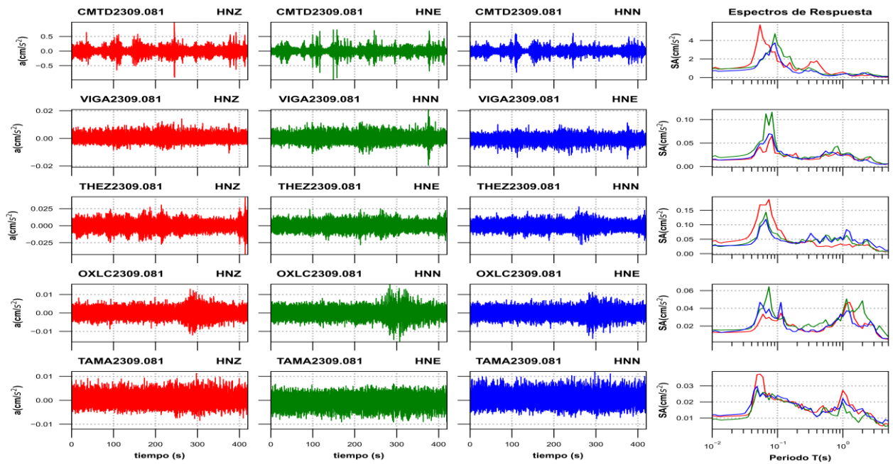
Figura 3f. Acelerogramas registrados y espectros de respuesta estimados para los registros obtenidos durante el sismo del 08 de septiembre de 2023 (M5.7)
