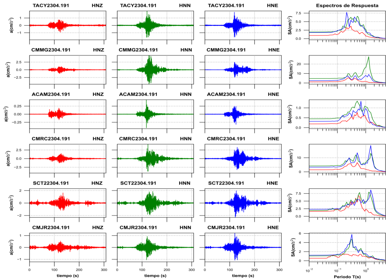
Figura 3c. Acelerogramas registrados y espectros de respuesta estimados para los registros obtenidos durante el sismo del 18 de abril de 2023 (M5.1)
