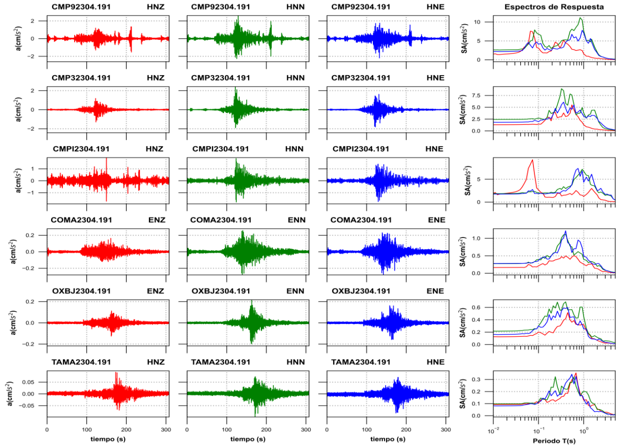
Figura 3f. Acelerogramas registrados y espectros de respuesta estimados para los registros obtenidos durante el sismo del 18 de abril de 2023 (M5.1)
