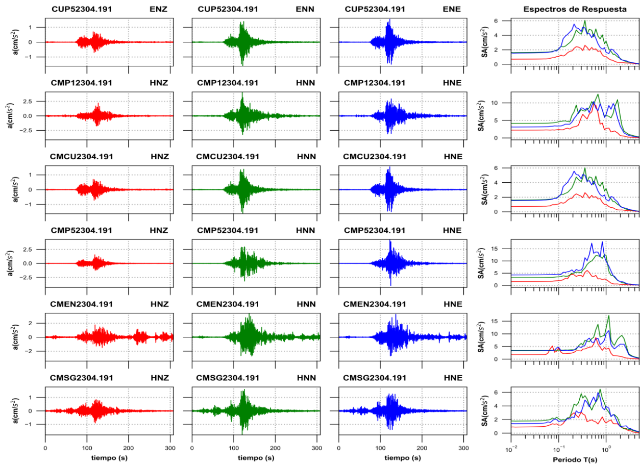
Figura 3b. Acelerogramas registrados y espectros de respuesta estimados para los registros obtenidos durante el sismo del 18 de abril de 2023 (M5.1)
