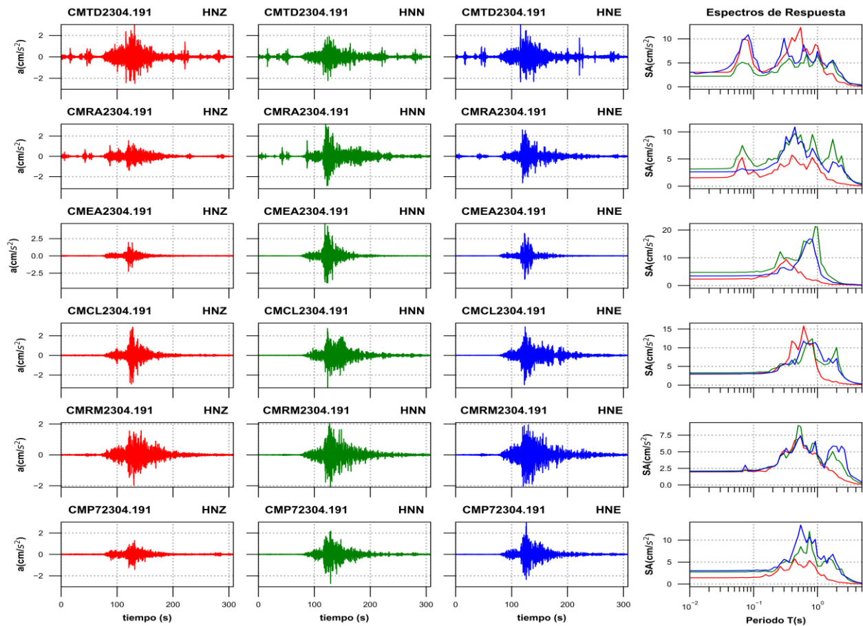
Figura 3d. Acelerogramas registrados y espectros de respuesta estimados para los registros obtenidos durante el sismo del 18 de abril de 2023 (M5.1)
