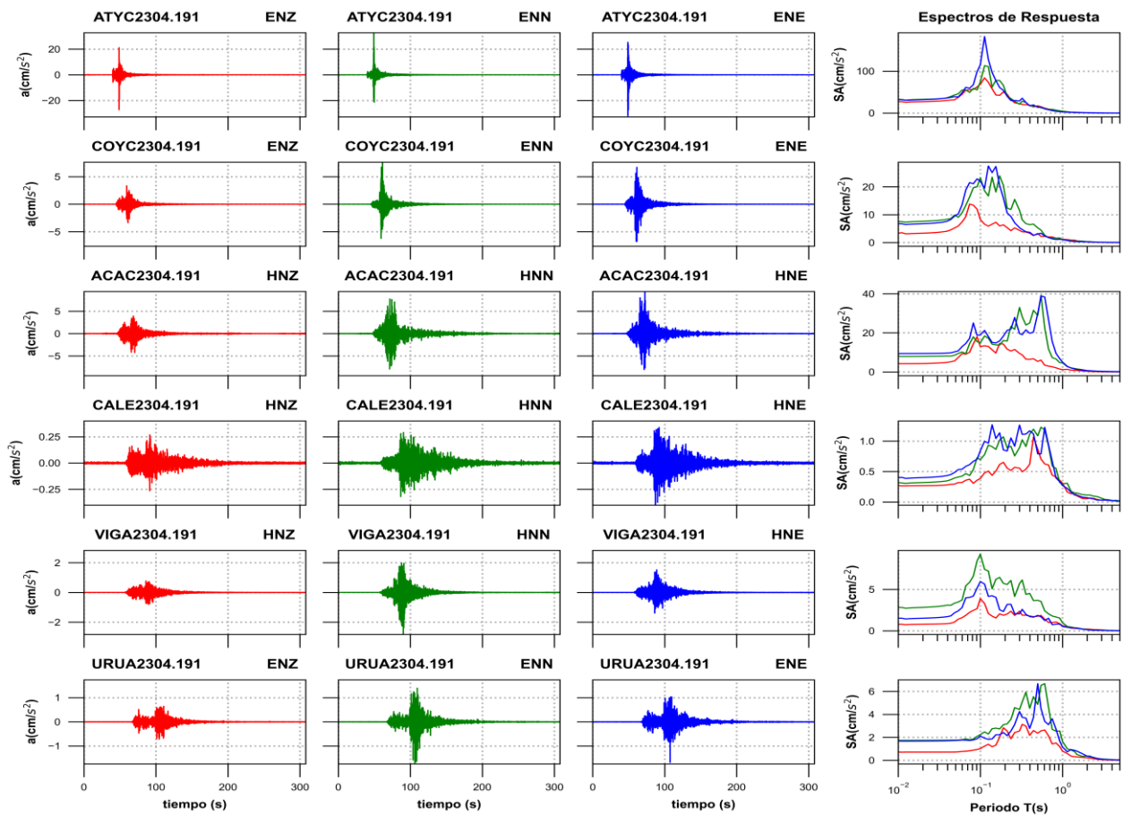
Figura 3a. Acelerogramas registrados y espectros de respuesta estimados para los registros obtenidos durante el sismo del 18 de abril de 2023 (M5.1)
