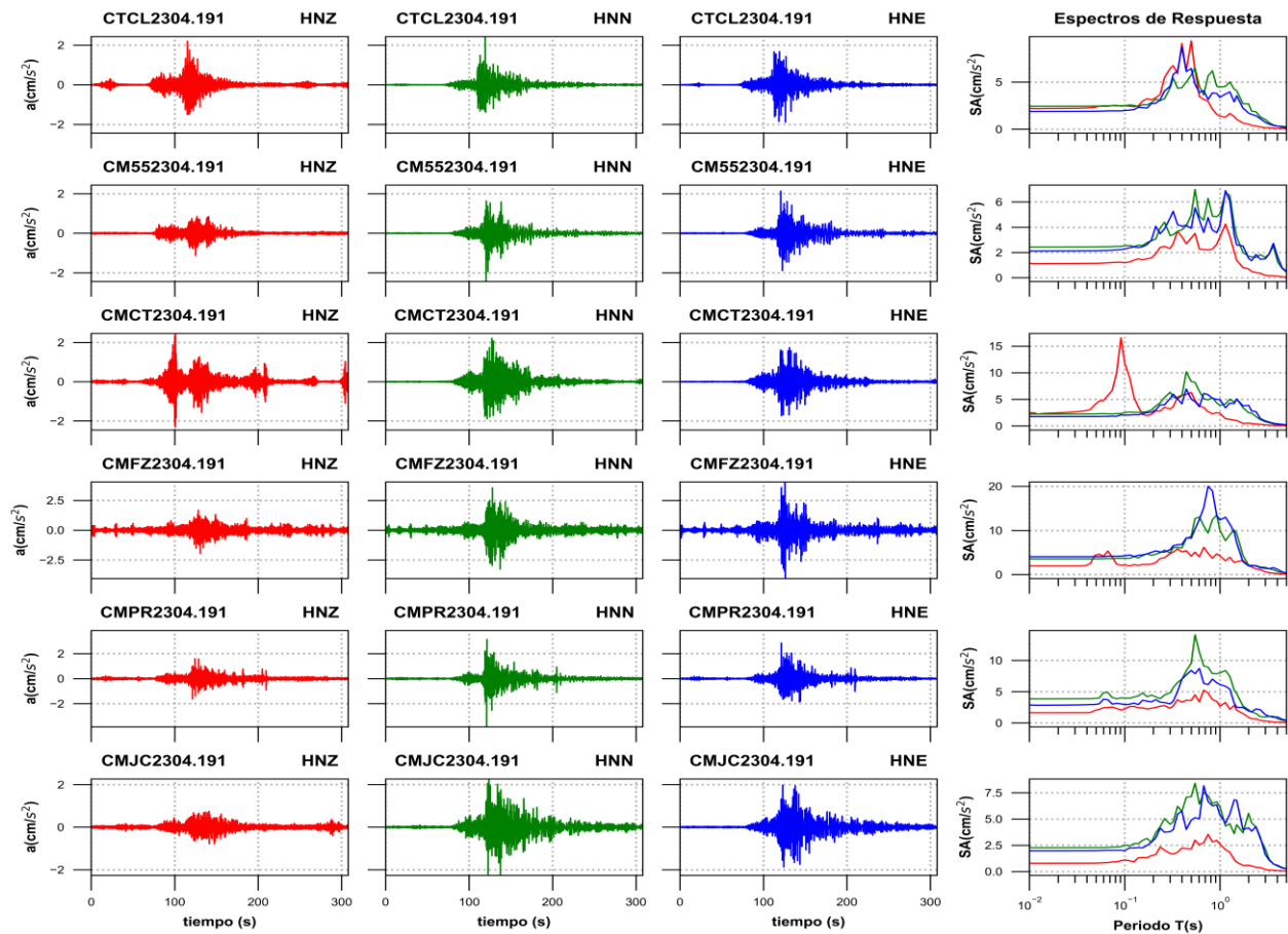
Figura 3e. Acelerogramas registrados y espectros de respuesta estimados para los registros obtenidos durante el sismo del 18 de abril de 2023 (M5.1)
