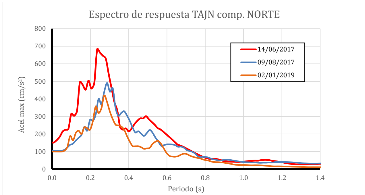
Figura 5. Espectros de respuesta estimados de la componente horizontal N registrados en la estación TAJN de los sismos del 14 de junio del 2017 (Mw6.9), 08 de septiembre de 2017 (Mw8.2) y 01 de febrero de 2019 (Mw6.5). Las respuestas espectrales fueron estimadas con el 5% de amortiguamiento.
