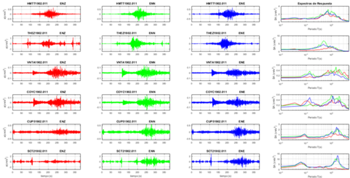
Figura 4b. Acelerogramas registrados y espectros de respuesta estimados para los registros obtenidos durante el sismo del 01 de febrero de 2019 (Mw6.5). Las componentes vertical (V), norte-sur (N) y este-oeste (E) corresponden a las líneas continuas en rojo, verde y azul, respectivamente.
