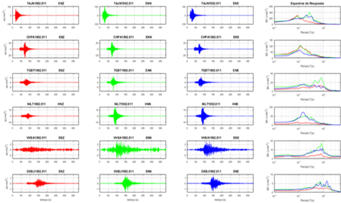
Figura 4a. Acelerogramas registrados y espectros de respuesta estimados para los registros obtenidos durante el sismo del 01 de febrero de 2019 (Mw6.5). Las componentes vertical (V), norte-sur (N) y este-oeste (E) corresponden a las líneas continuas en rojo, verde y azul, respectivamente.
