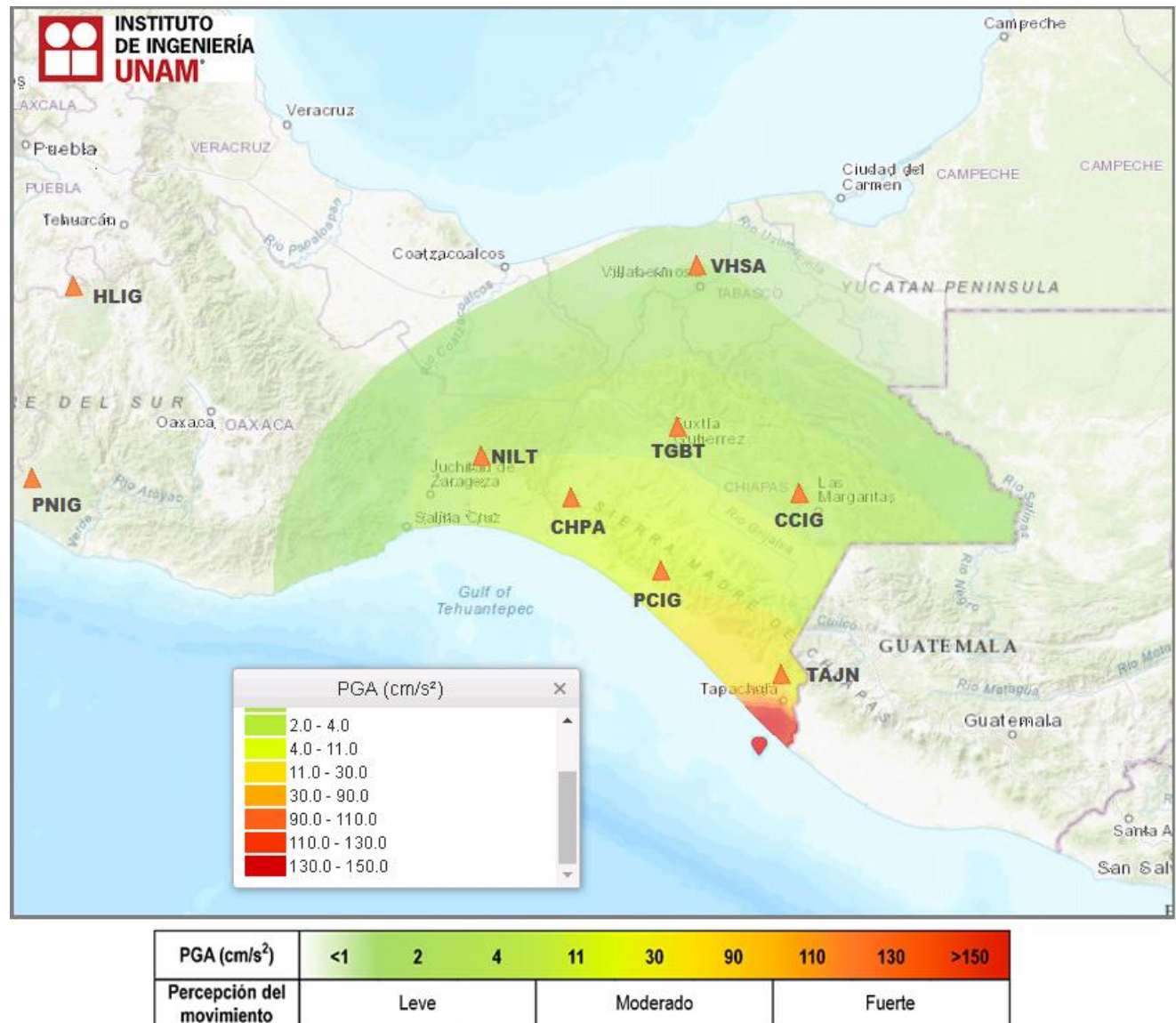
Figura 2. Mapa de Intensidad PGA_{rmsh} . Media cuadrática de las aceleraciones pico horizontales.
